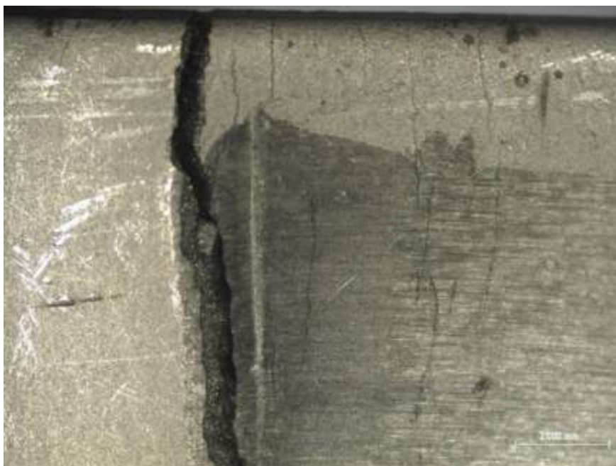
Slika 93. Pukotina na vanjskoj površini luka uzorka od čelika EN 1.4301 (AISI 304).
