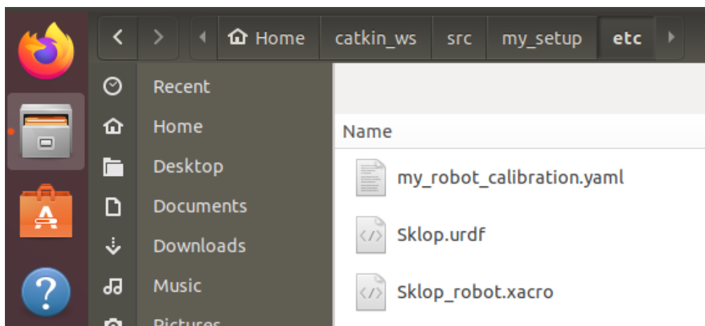
Slika 13. My_setup direktorij
