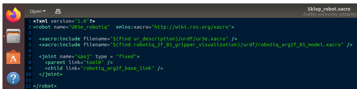
Slika 14. etc direktorij
