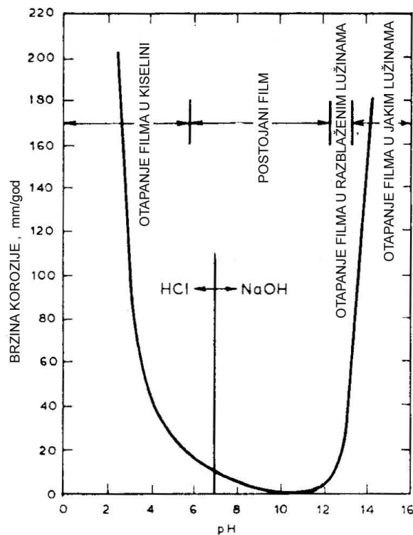
Slika 5. Utjecaj pH na brzinu korozije cinka
