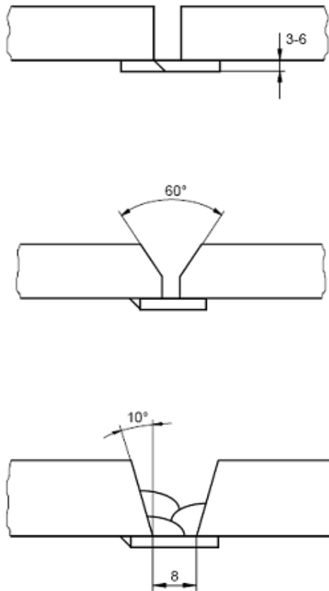
Slika 5. Oblici metalnih podloška [2]
