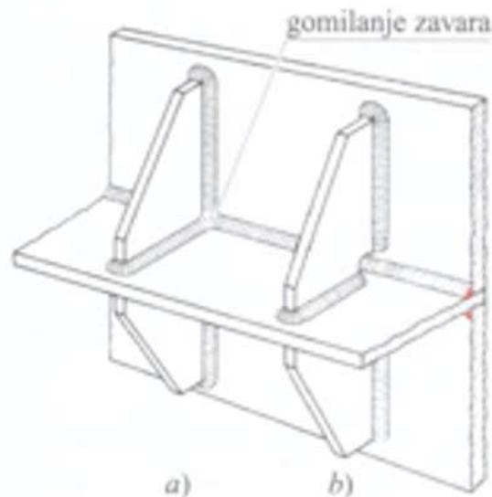
Slika 13 Privarena rebra
