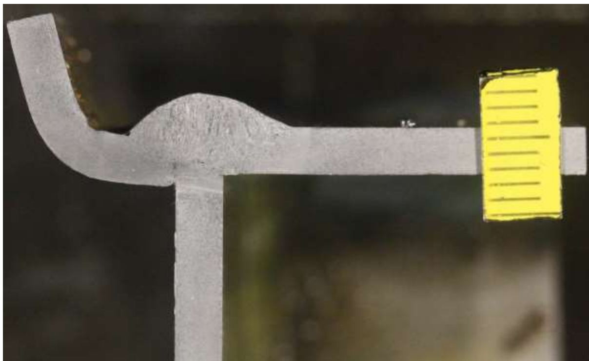
Slika 39 Uzorak 1, presjek 1
