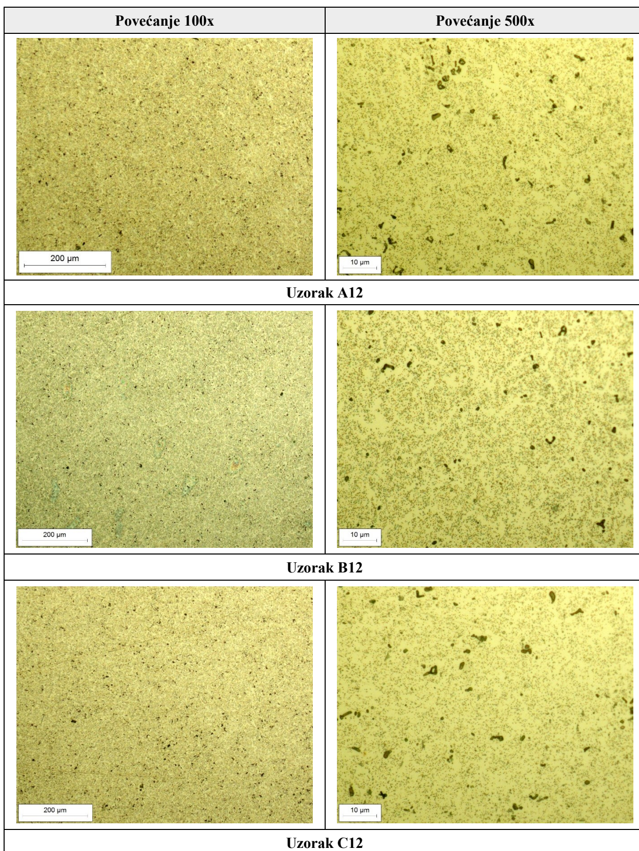
Tablica 6.11 Mikrostruktura uzoraka A12, B12 i C12
