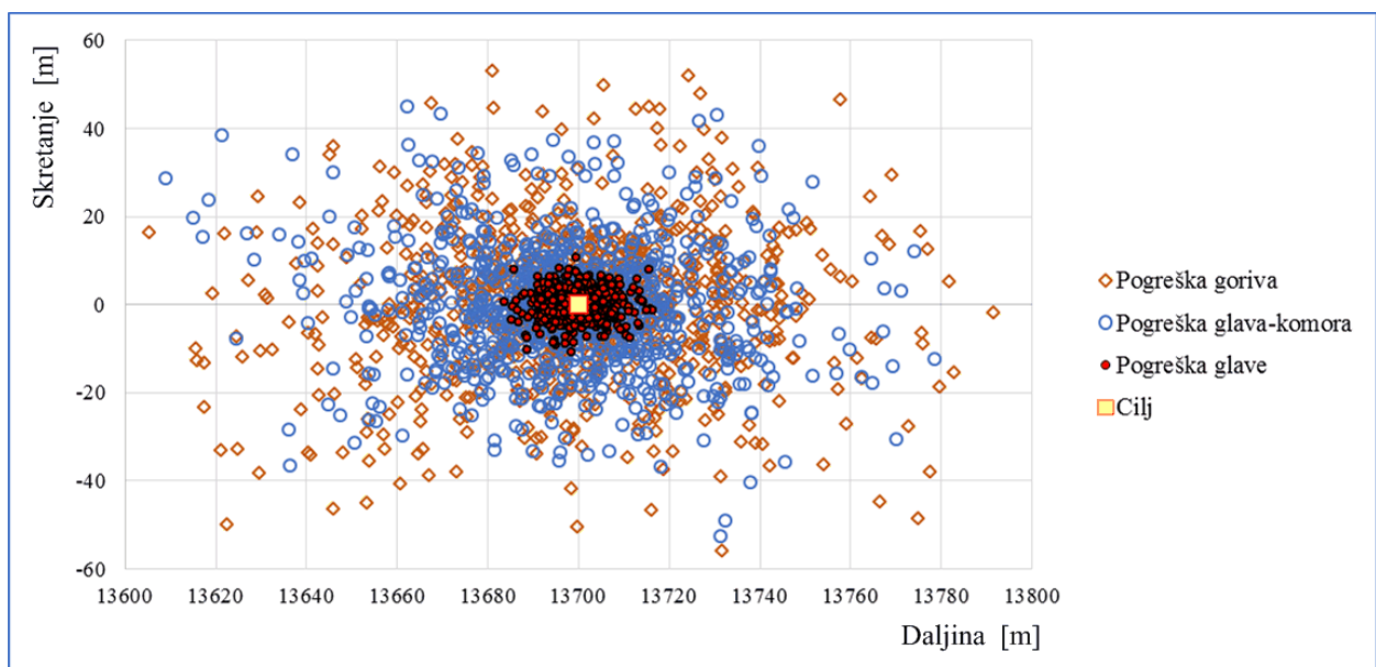
Slika 6.27. Usporedba disperzije padnih točaka zbog pogrešaka \delta_P , odnosno \delta_{HC} i \delta_H
