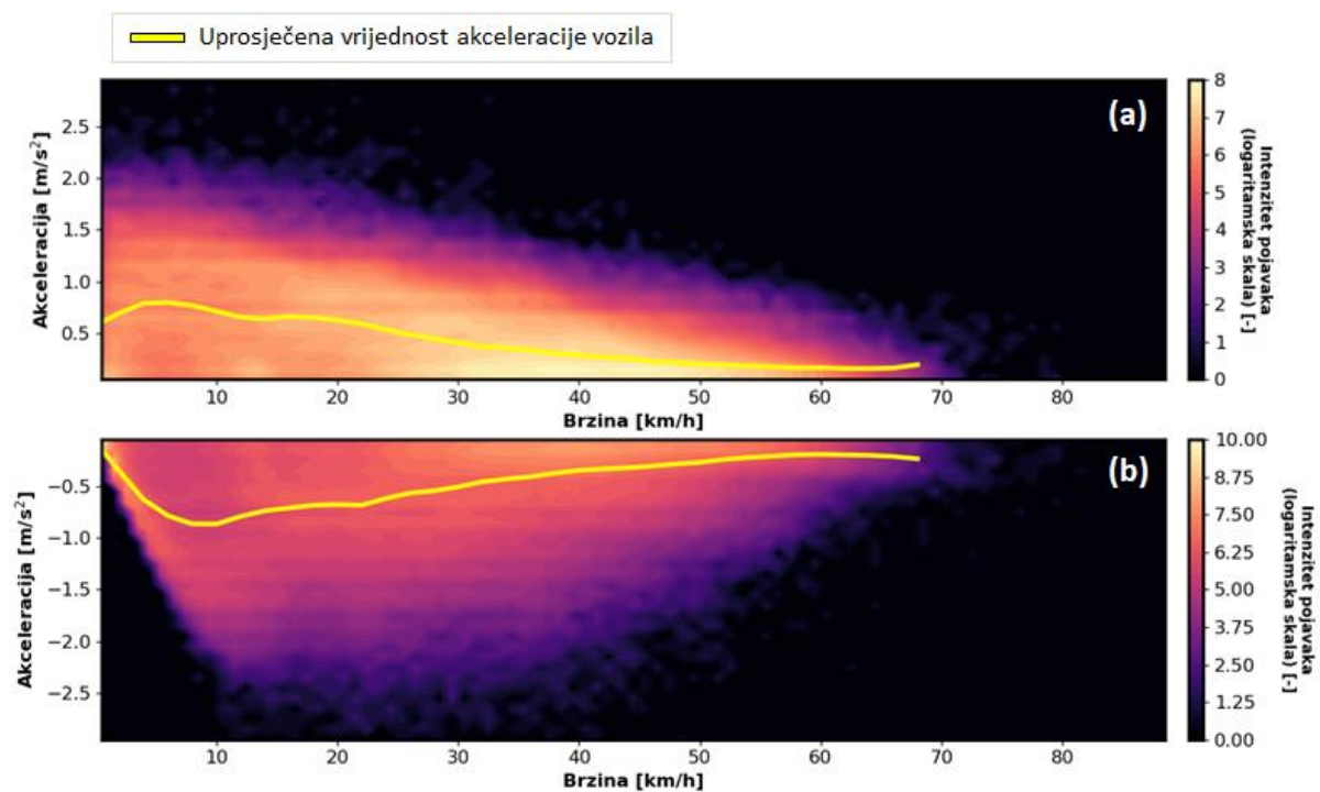
Slika 2-13: Toplinske mape a) pozitivnog i b) negativnog ubrzanja vozila s obzirom na brzinu vozila za objedinjenu rutu BK-P-BK, uključujući po brzini uprosječne vrijednosti ubrzanja vozila.
