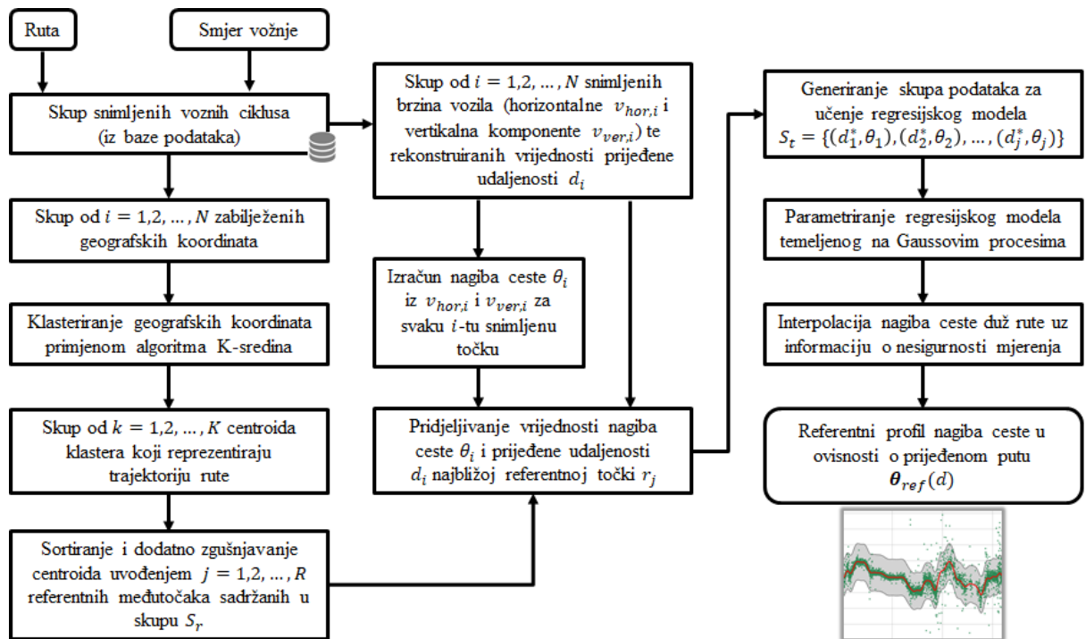
Slika 2-5: Blokovski dijagram metode rekonstrukcije profila nagiba ceste duž rute temeljem snimljenih GPS podataka vožnje.
