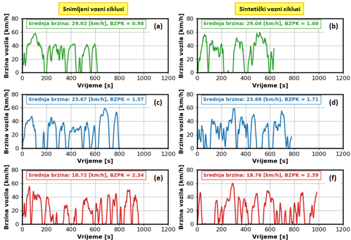
Slika 3-12: Reprezentativni primjeri vremenskih profila brzine vozila za a), c), e) snimljene i b), d), f) sintetičke vozne cikluse dobivene za klastere lagane (zelena boja), srednje (plava boja) i teške zagušenosti prometa (crvena boja). Oznaka BZPK odnosi se na broj zaustavljanja vozila po kilometru.
