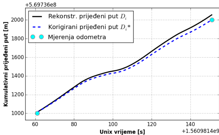
Slika 2-2: Primjer GPS-rekonstruiranog D_i i temeljem odometra-korigiranog D_i^* profila prijednog puta između dva susjedna mjerenja odometra.
