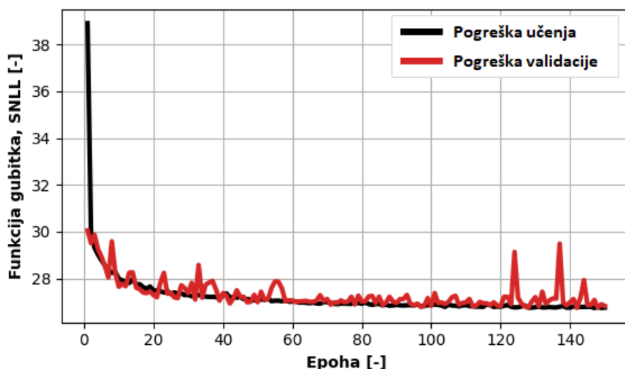
Slika 7-21: Krivulje pogreške učenja i validacije kroz epohe učenja za NN-DSTC model.
