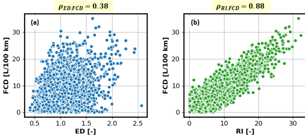
Slika 6-5: Ovisnosti pokazatelja odstupanja potrošnje goriva (FCD) o pokazateljima reprezentativnosti voznih ciklusa a) ED i b) RI za slučaj 3000 sintetičkih voznih ciklusa, uključujući pripadne vrijednosti indeksa korelacije ( \rho_{ED,FCD} , \rho_{RI,FCD} ).
