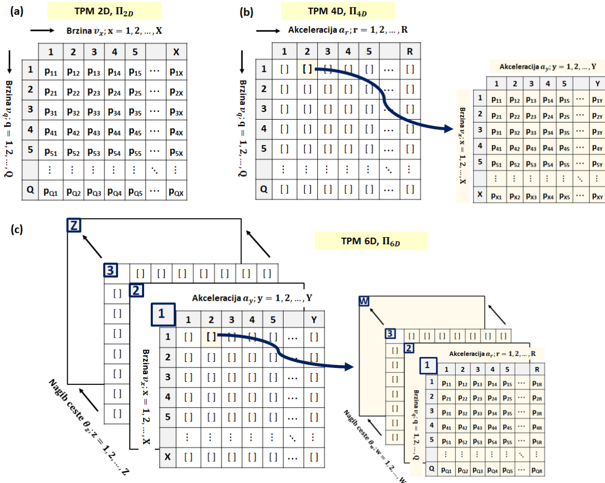
Slika 3-4: Ilustracija a) 2D , b) 4D i c) 6D TPM-a implementiranog u obliku niza.
