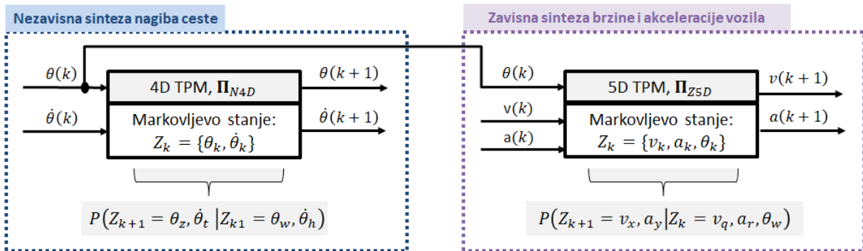
Slika 3-3: Koncept modela temeljenog na hijerarhijskoj sintezi voznih ciklusa (ML-HIER) koji se sastoji od nezavisne \Pi_{N4D} i zavisne \Pi_{Z5D} matrice prijelaznih vjerojatnosti.
