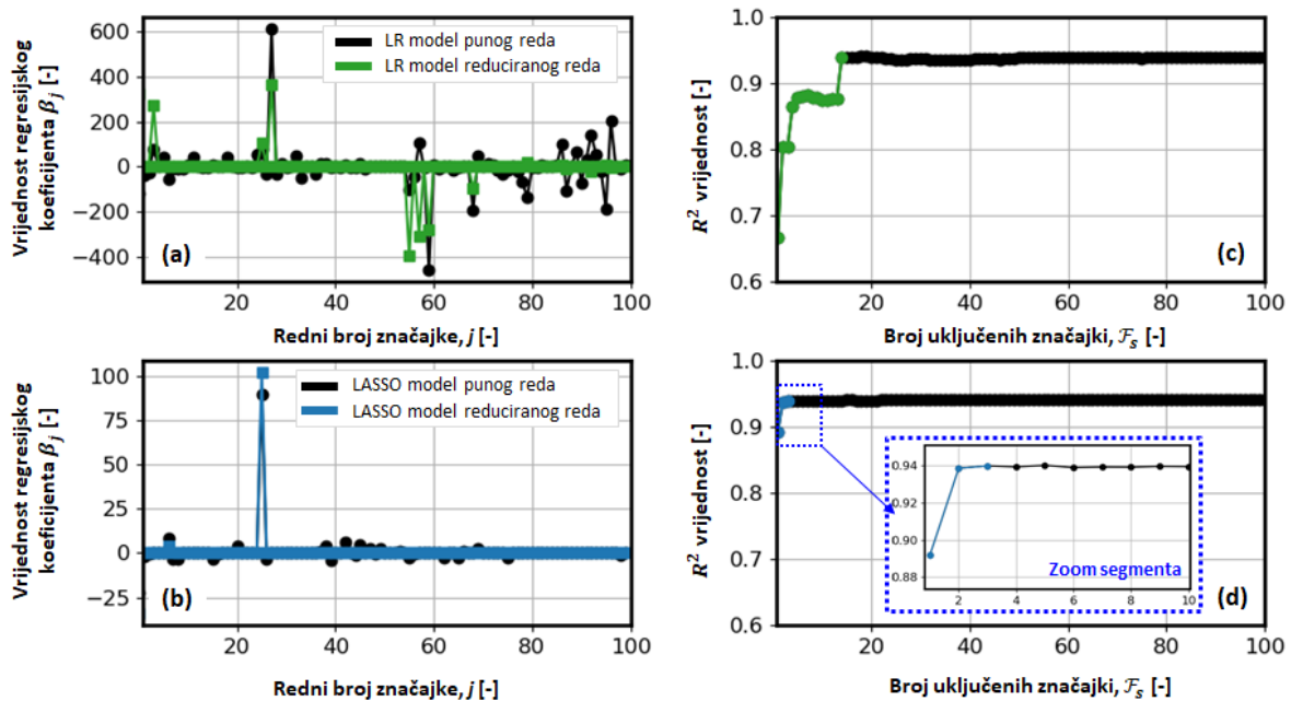
Slika 6-4: Vrijednosti koeficijenata regresije \hat{\beta}_j za slučaj a) LR i b) LASSO modela punog i reduciranog reda; te postignute R^2 vrijednosti c) LR i d) LASSO modela u ovisnosti o broju ulaznih značajki tj. parametara.
