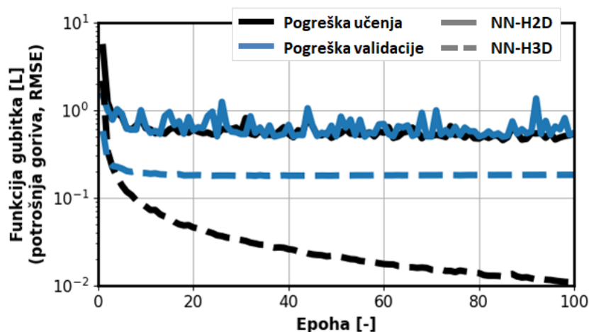
Slika 4-11: Krivulje pogreške učenja i validacije kroz epohe učenja za NN-H2D (puna linija) i NN-H3D (isprekidana linija).
