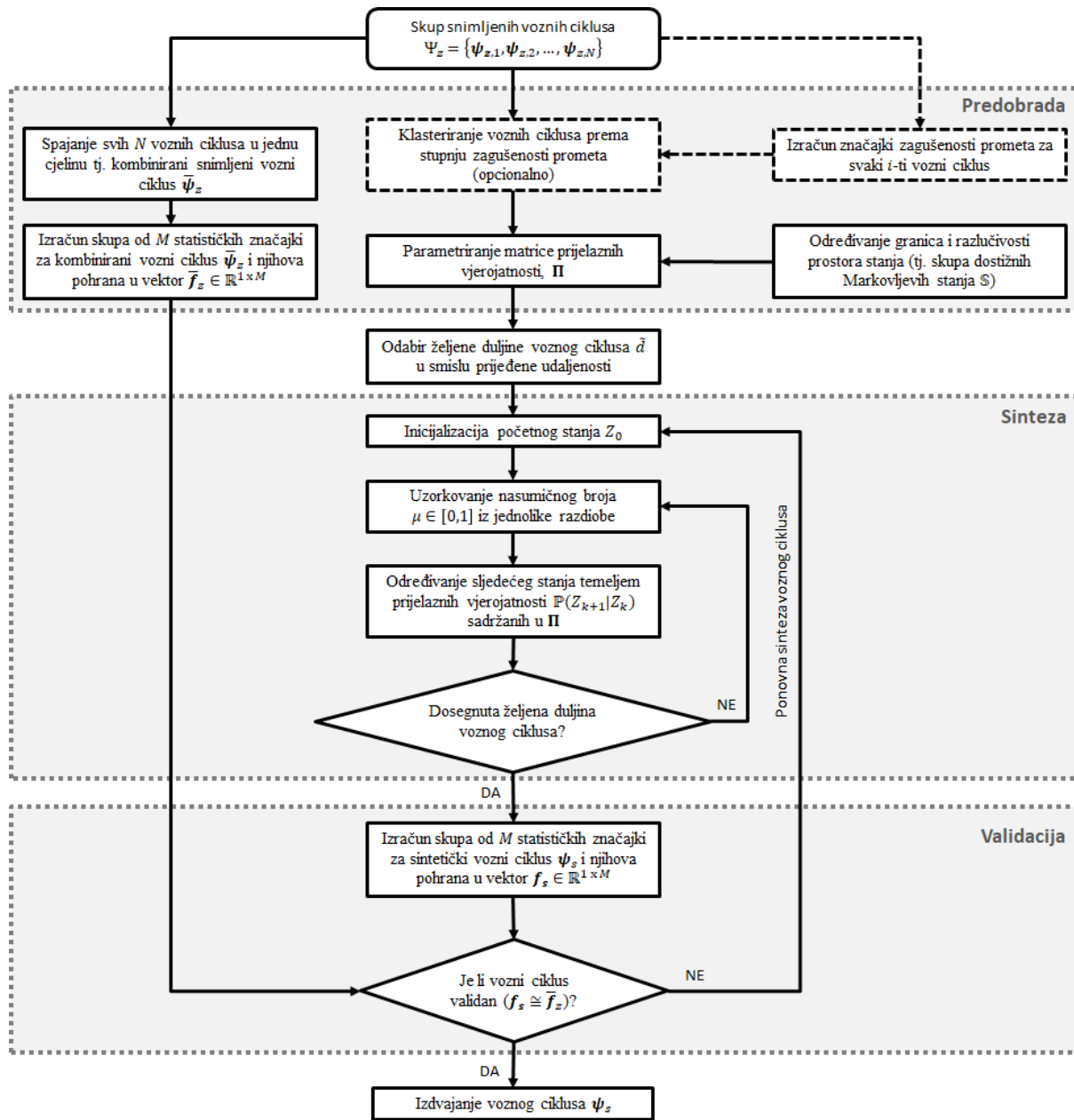
Slika 3-1: Blokovski dijagram metode sinteze vozničkih ciklusa temeljene na Markovljevim lancima, uključujući osnove validacije vozničkih ciklusa.
