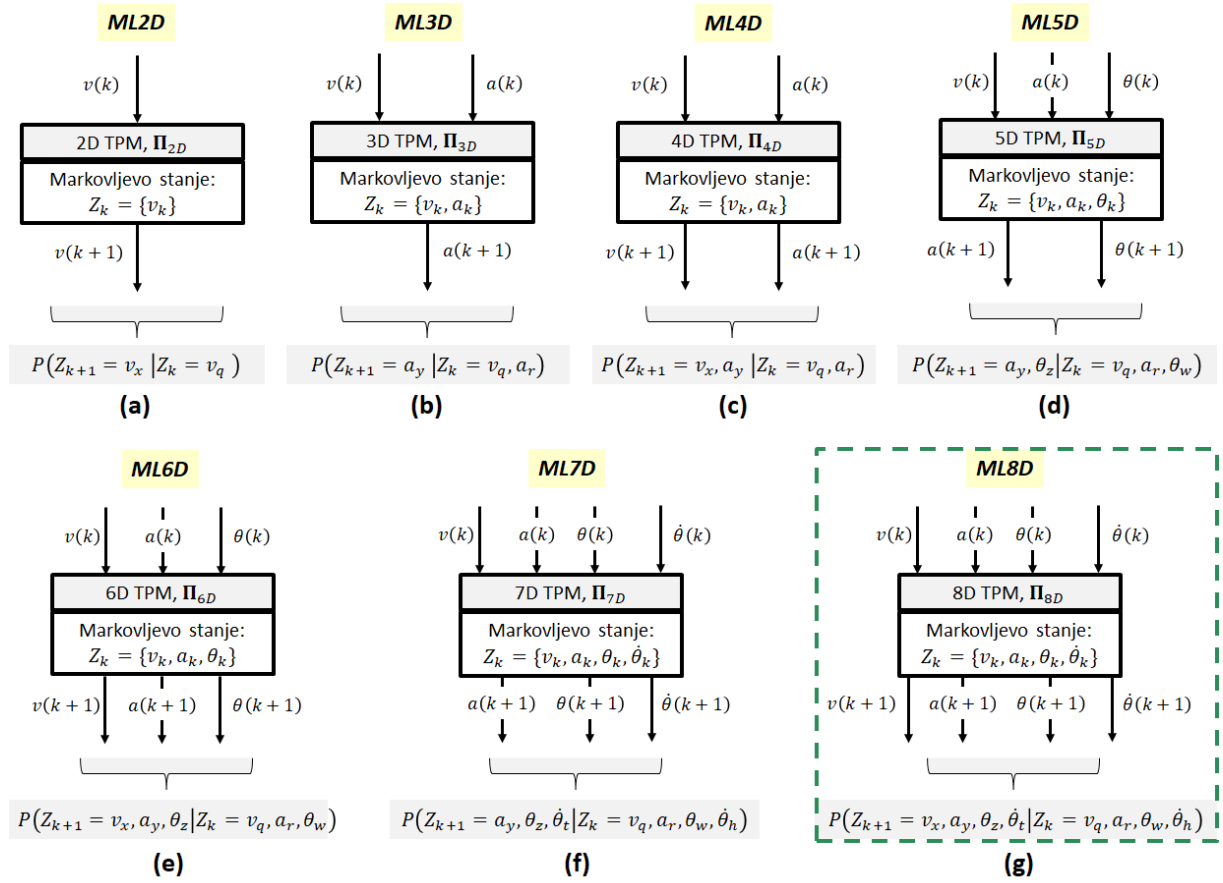
Slika 3-2: Prikaz različitih koncepata (modela) realizacije Markovljevog lanca u smislu dimenzionalnosti matrice prijelaznih vjerojatnosti \Pi .
