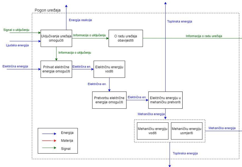
Slika 24. Pogon uređaja
