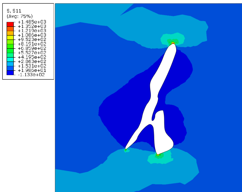
Slika 29 Dijagram naprezanja \sigma_x /MPa modela 1 visoke kompleksnosti
