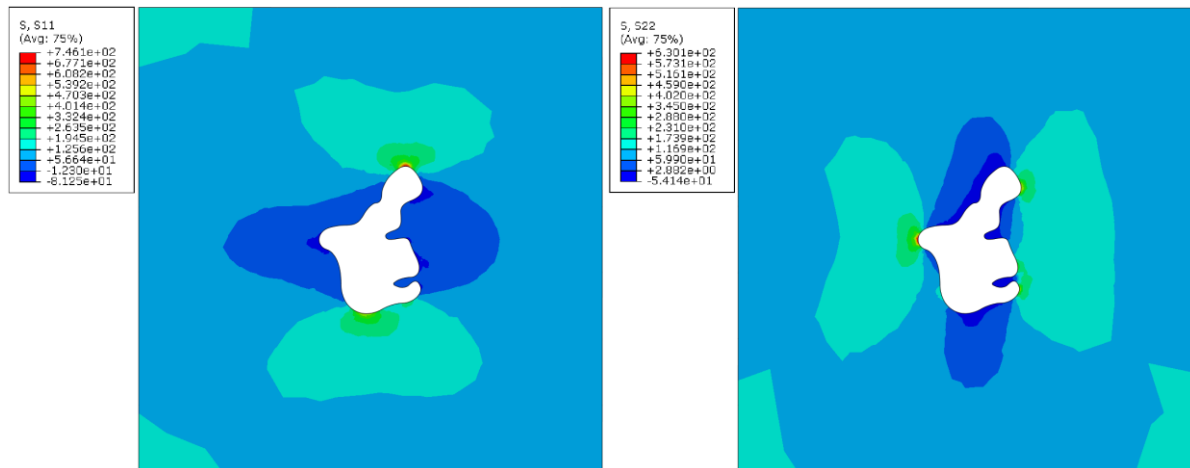
Slika 39 Dijagram naprezanja \sigma_x /MPa (lijevo) i \sigma_y /MPa (desno) za model 4 srednje kompleksnosti
