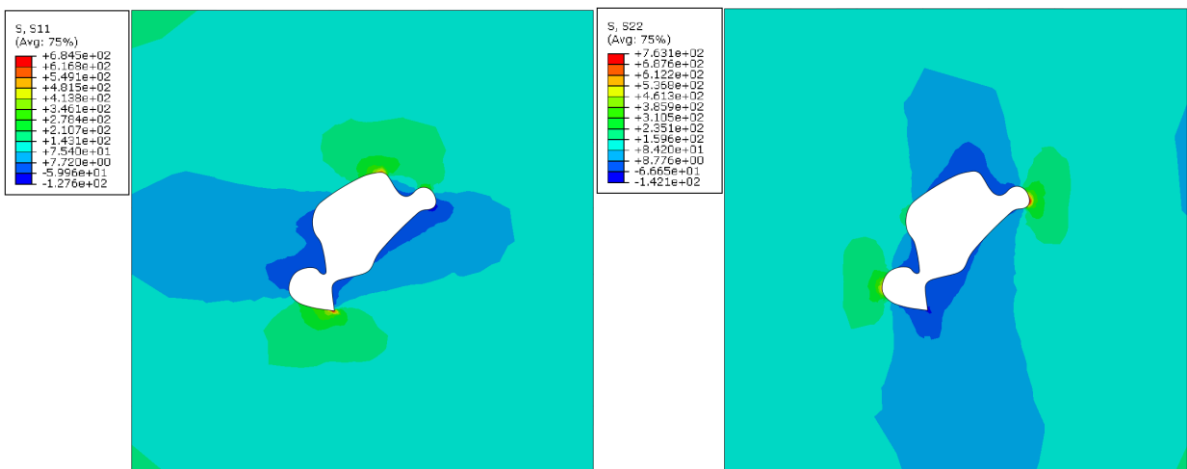
Slika 37 Dijagram naprezanja \sigma_x /MPa (lijevo) i \sigma_y /MPa (desno) za model 2 srednje kompleksnosti
