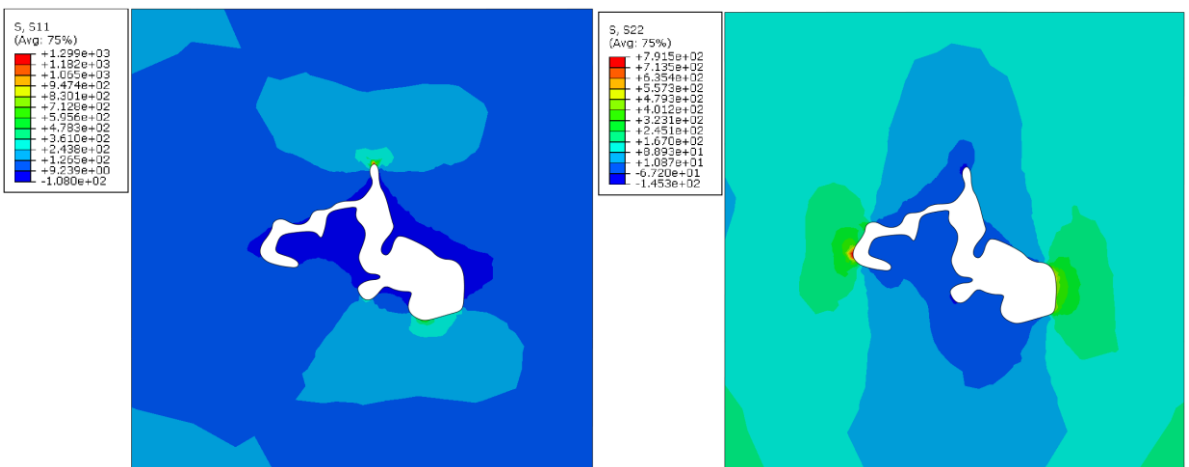
Slika 43 Dijagram naprezanja \sigma_x /MPa (lijevo) i \sigma_y /MPa (desno) za model 4 visoke kompleksnosti
