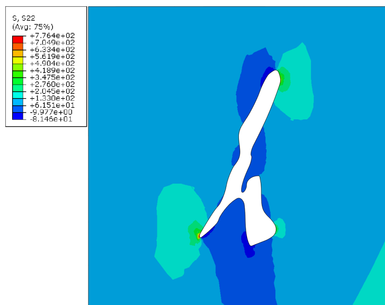
Slika 30 Dijagram naprezanja \sigma_y /MPa modela 1 visoke kompleksnosti
