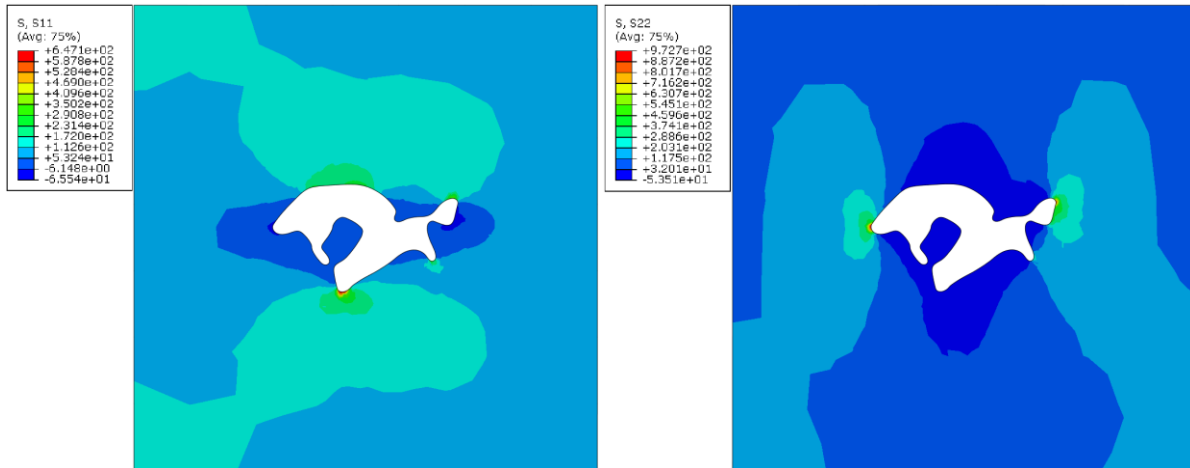
Slika 38 Dijagram naprezanja \sigma_x /MPa (lijevo) i \sigma_y /MPa (desno) za model 3 srednje kompleksnosti
