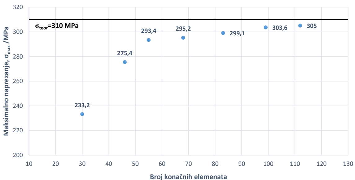
Slika 13 Konvergencija naprezanja u odnosu na broj elemenata kod pore kružnog oblika
