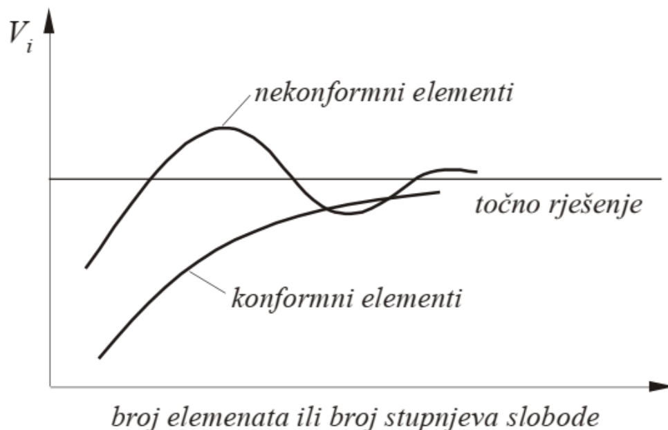
Slika 10 Konvergencija rješenja [9]
