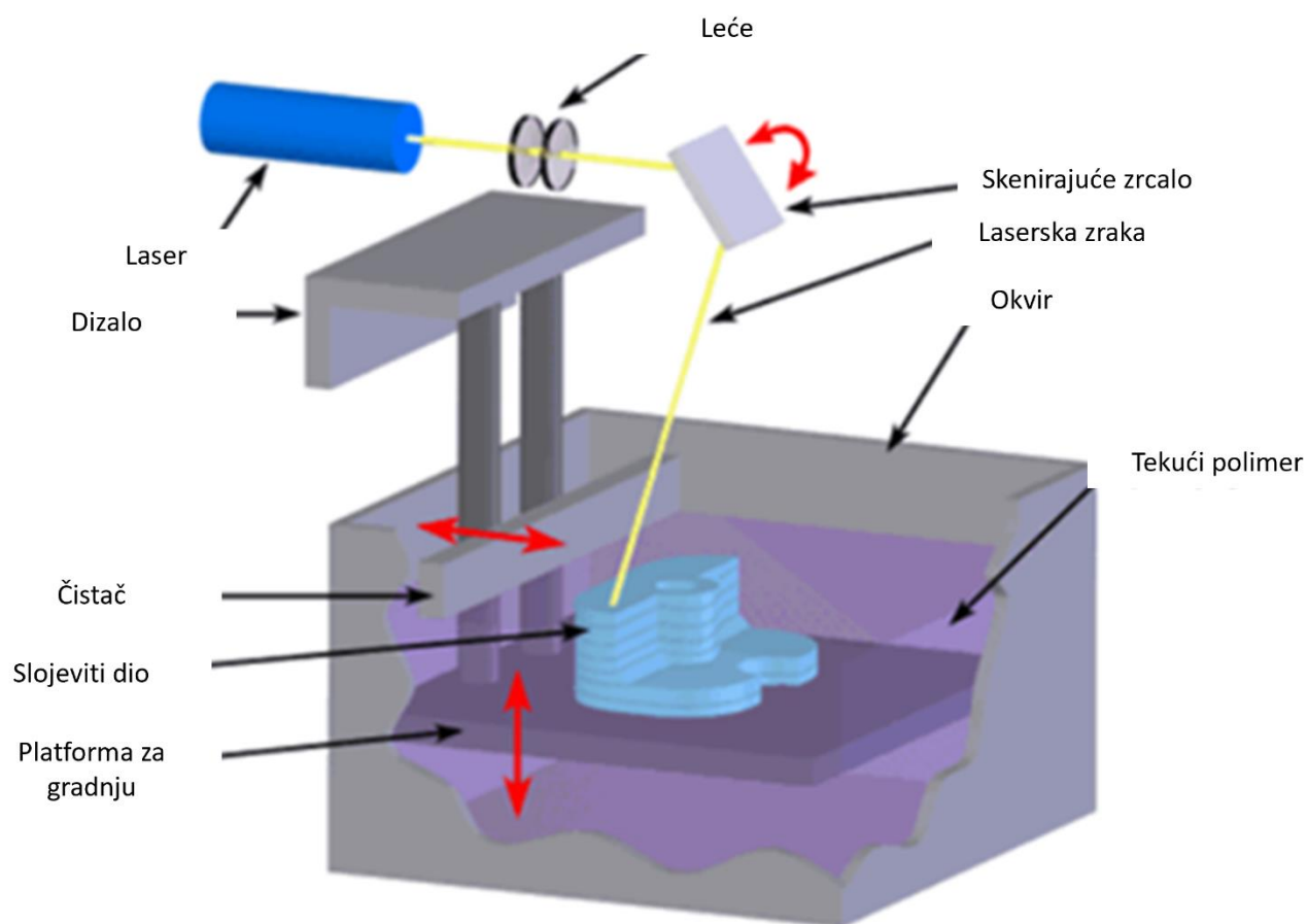
Slika 4. Stereolitografija [5]
