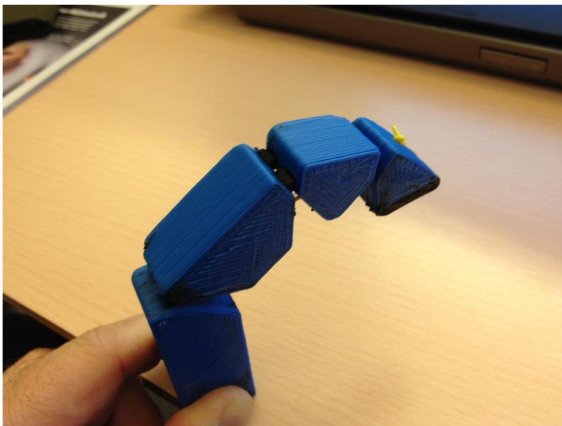
Slika 19. Proteza prsta izrađena vodljivim filamentom [24]
