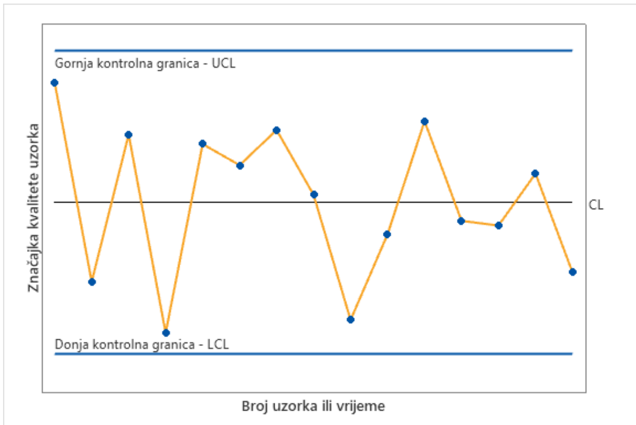
Slika 5. Kontrolna karta
