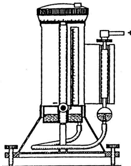
Slika 8. Minimetar [3]
