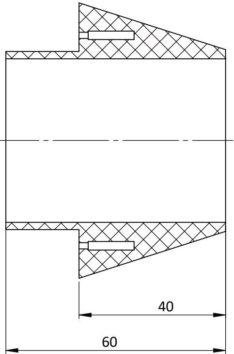
Presjek B-B:
