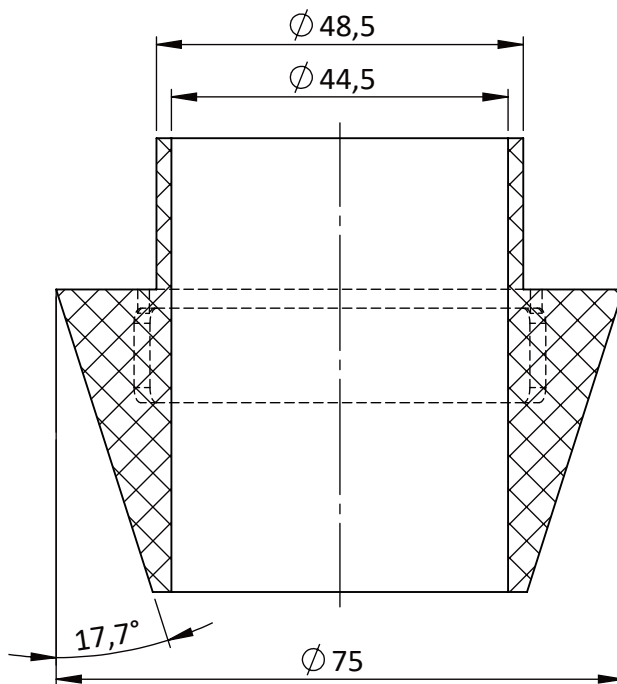
Presjek A-A:
