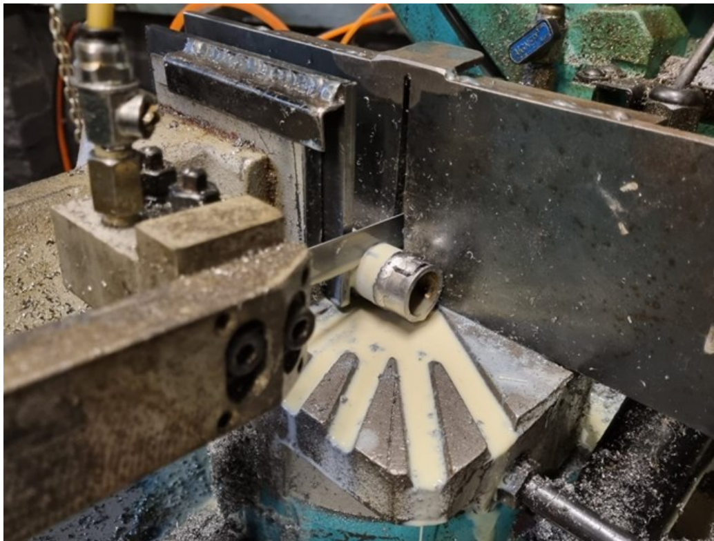
Slika 30. Postupak rezanja cijevi tračnom pilom
