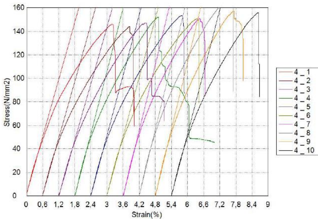
Slika 24. Graf naprezanje - istežanje kod savojnog ispitivanja (četiri sloja vlakana)
