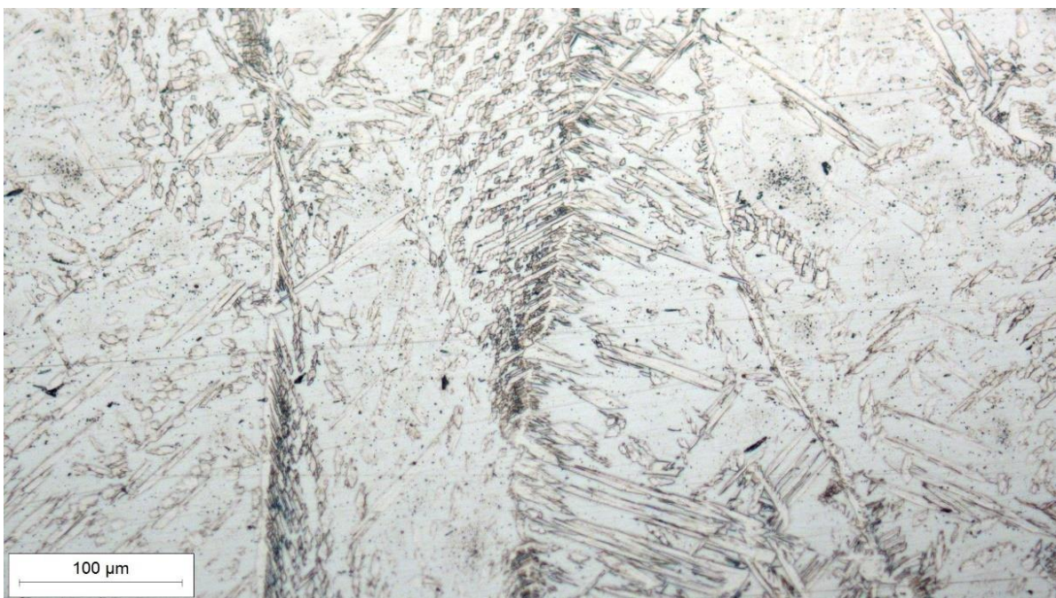
Slika 37. Mikrostruktura navara uzorka 1A uz povećanje 200x
