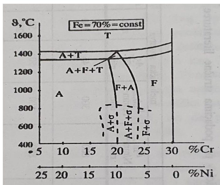
Slika 11. Kvazibinarni dijagram stanja duplex čelika uz 70% Fe = const [7]
