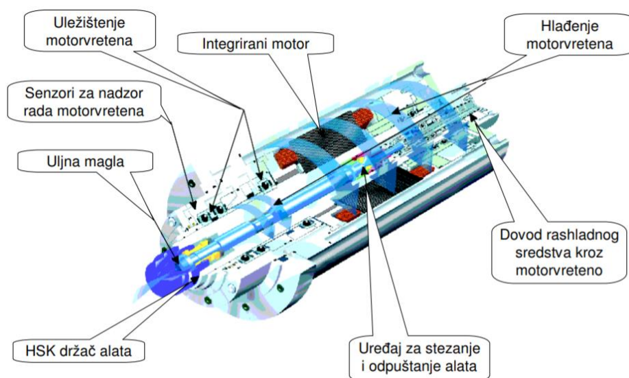
Slika 7. Motorvreteno [1]
