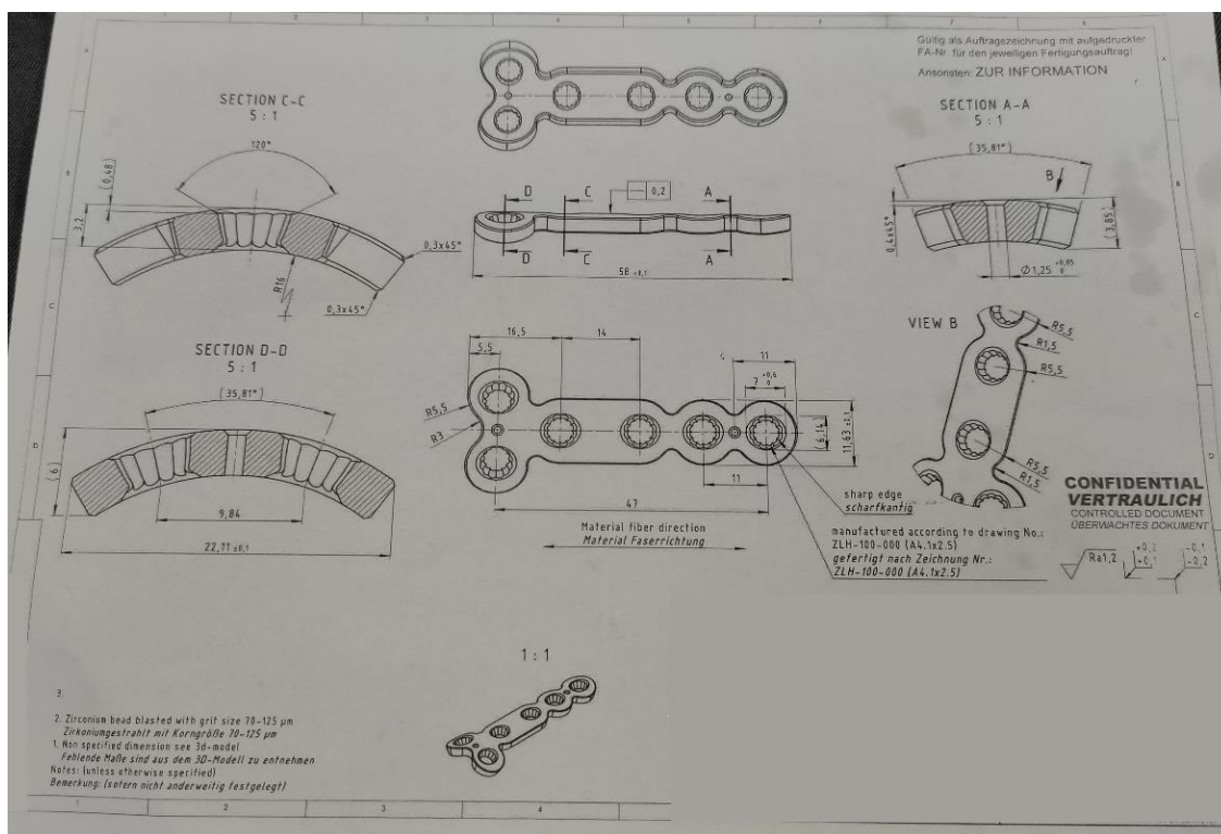
Slika 27. Konstrukcijski nacrt pločice
