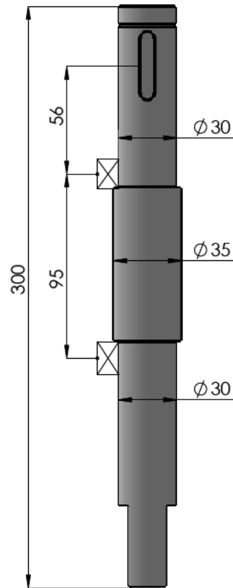
Slika 16. Skica vratila V2
