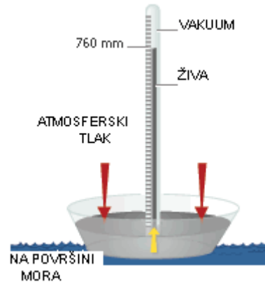
Slika 2 - Torricelliev barometar
