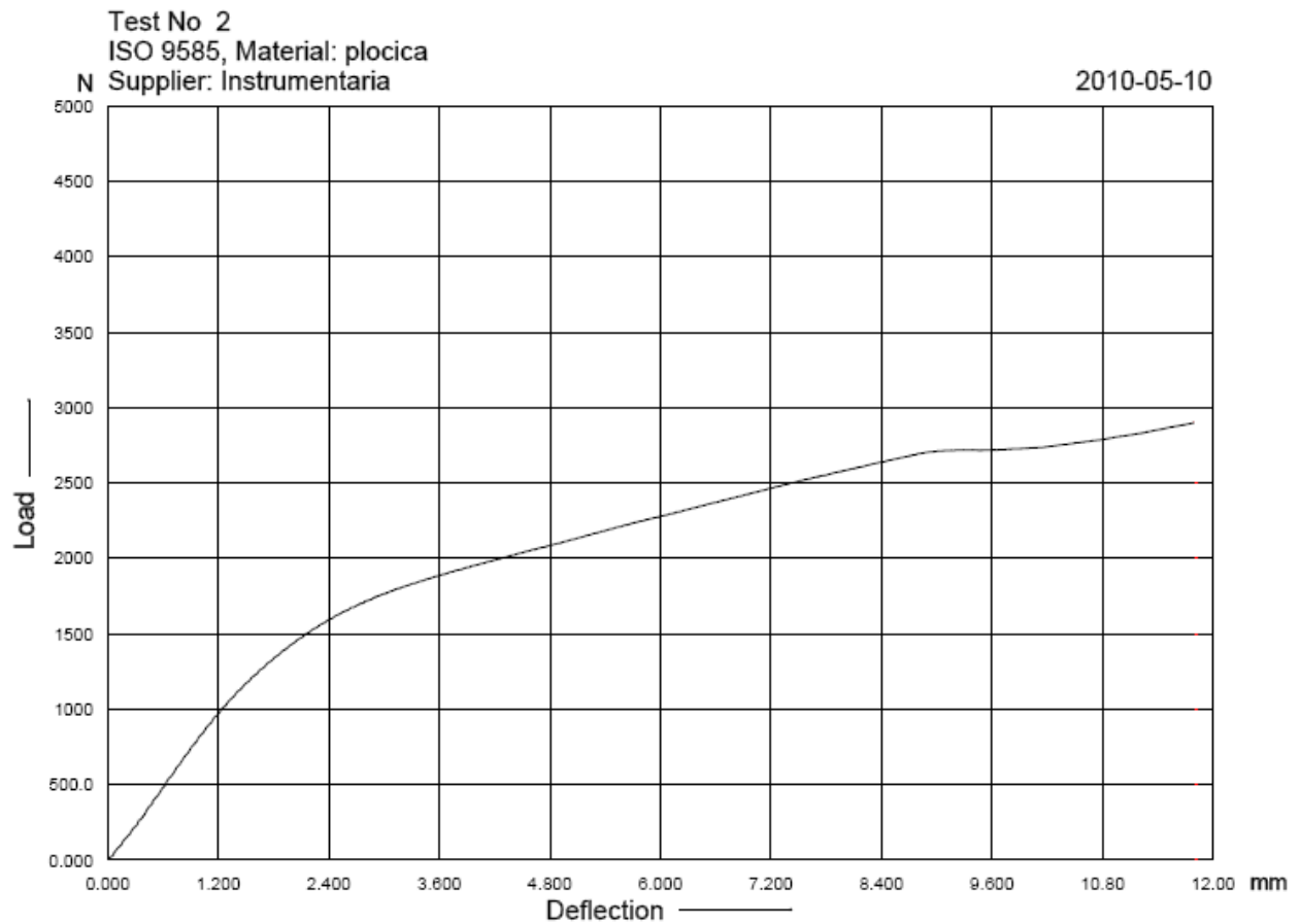
Slika 5.10 Dijagram sila-progib za poprečno ožljebljenu pločicu
