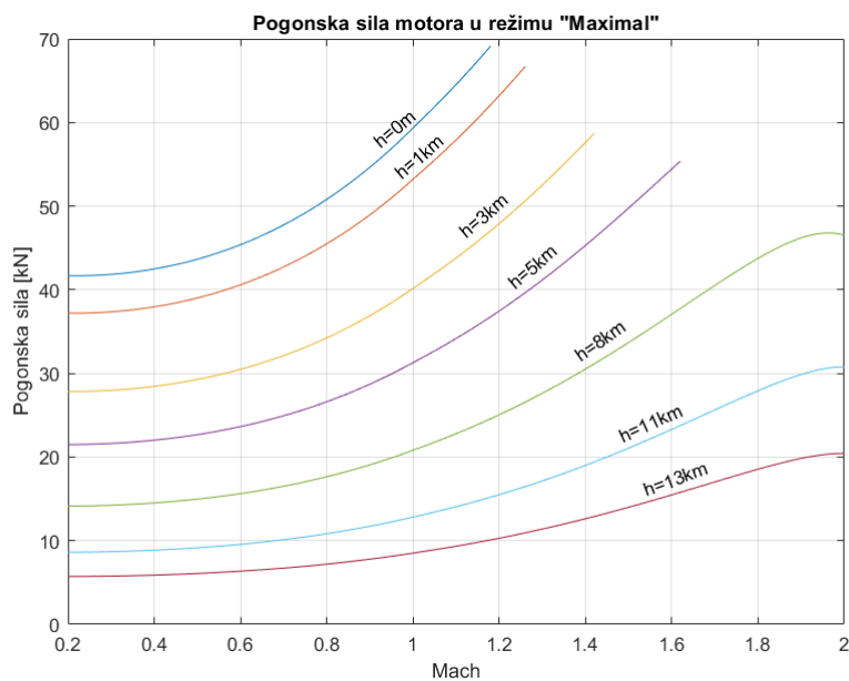
Slika 4.3: Pogonska sila motora u režimu "Maximal"
