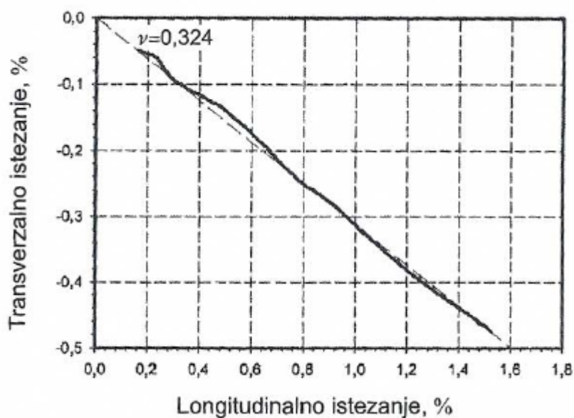
Slika 18. Odnos transverznog i longitudinalnog istežanja [9]
