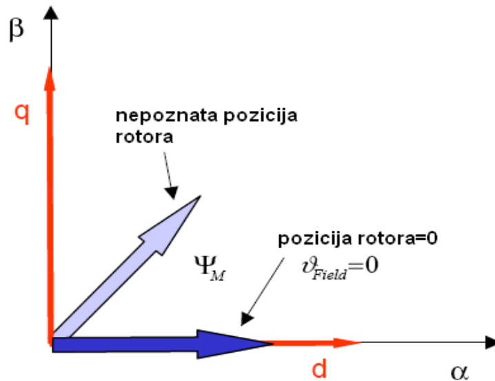
Slika 33. Namještanje rotora [19]
