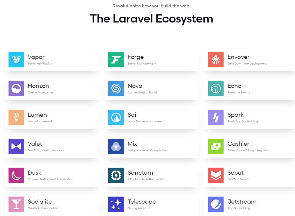
Slika 8. Laravel ekosustav[8]
