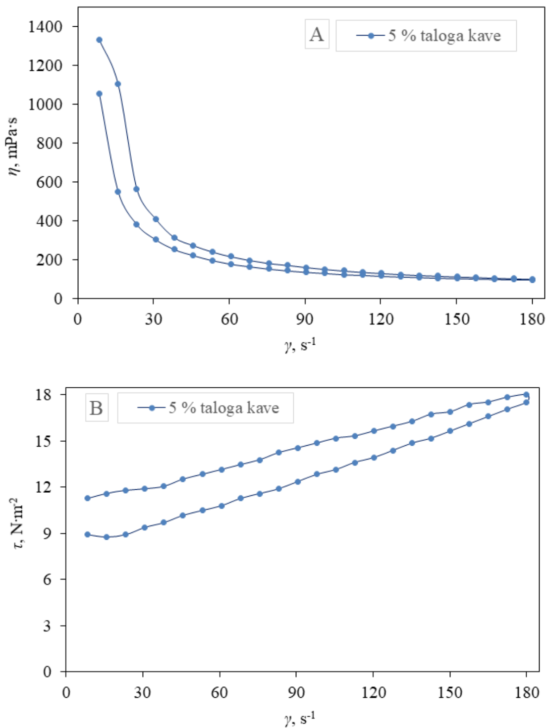
Slika 28. Krivulje tečenja 60 %-tnih suspenzija (sustav s 95 % Al 2 O 3 i 5 % otpadnog taloga kave): (A) ovisnost providne viskoznosti ( \eta , mPa·s) o brzini smicanja ( \gamma , s -1 ), (B) ovisnost smičnog naprezanja ( \tau , N·m -2 ) o brzini smicanja ( \gamma , s -1 )
