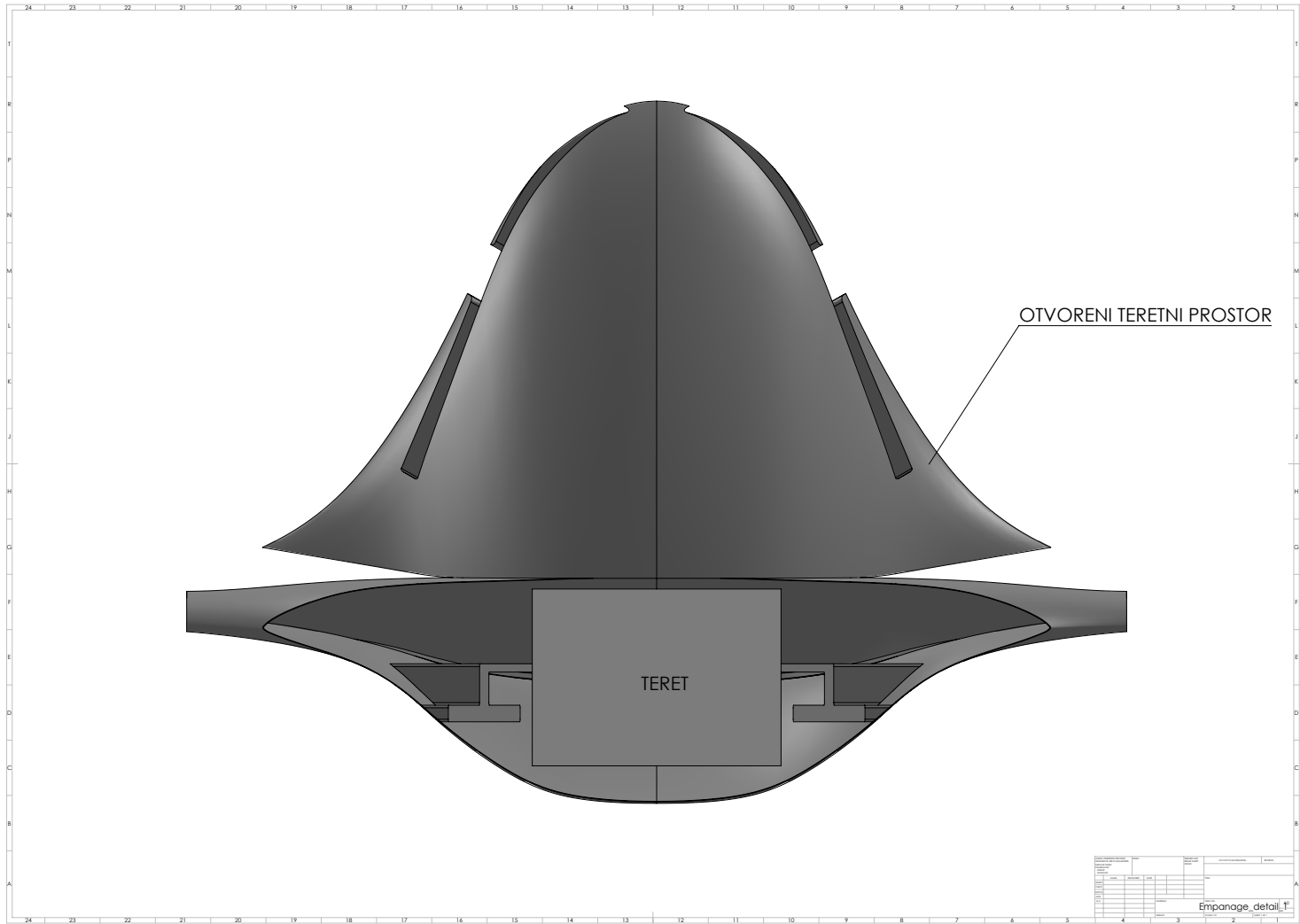
Slika B.3: Nacrt trupa letjelice
