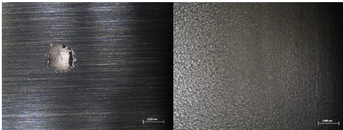
Slika 22. Usporedba površine austenitnog čelika EN 1.4404 (AISI 316L) i superaustenitnog čelika EN 1.4539 (AISI 904L) nakon korozijskog ispitivanja na 20 °C
