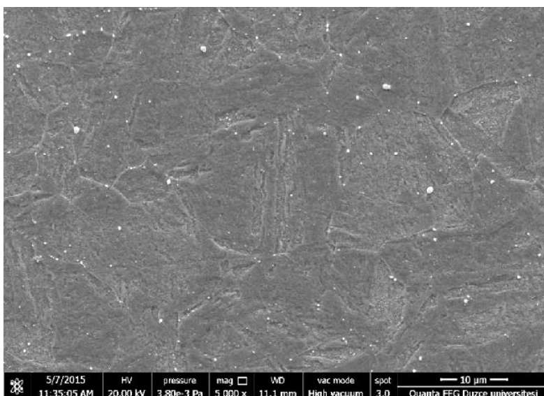
Slika 7. Mikrostruktura precipitacijski očvrsnutog nehrđajućeg čelika [12]
