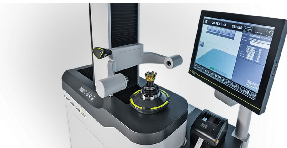
Slika 36. Uređaj za prednamještanje alata Zoller
