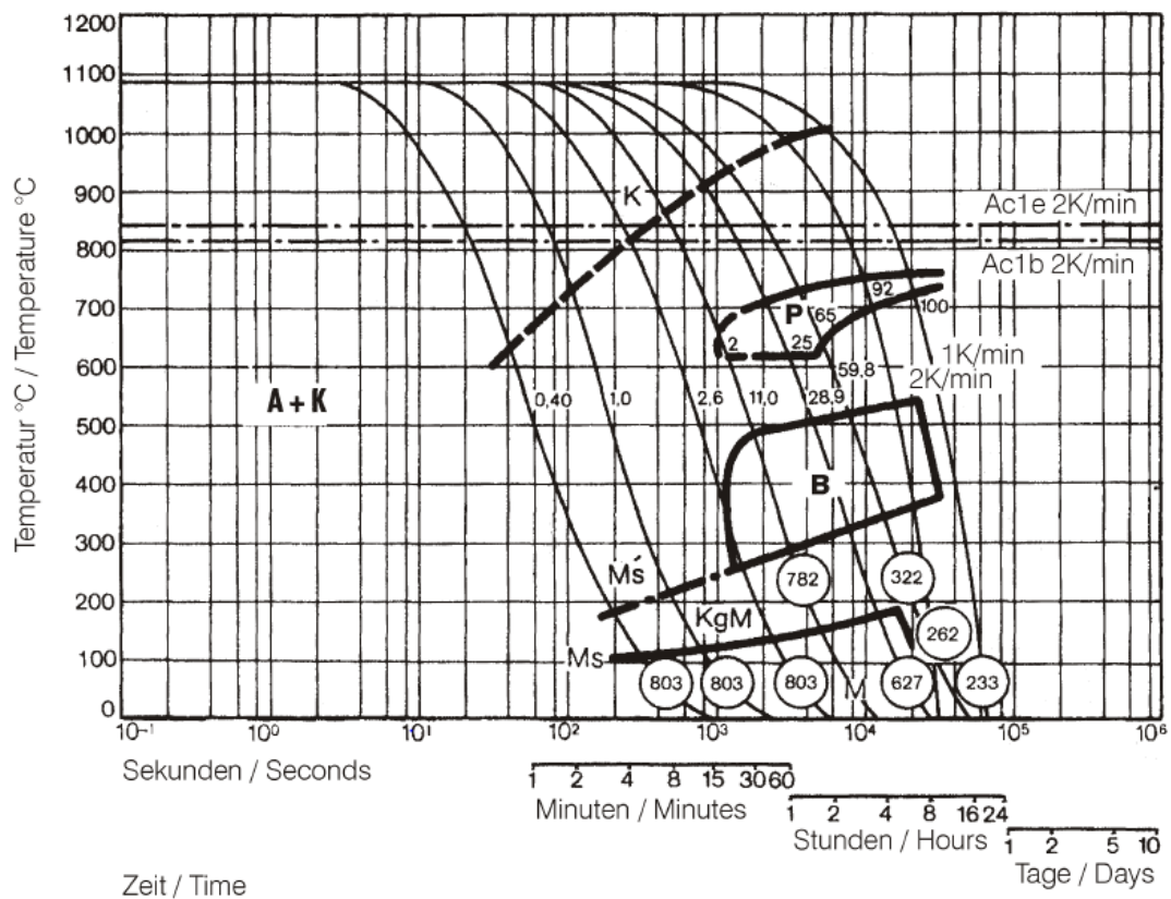
Slika 33. TTT dijagram – K110DE [26]
