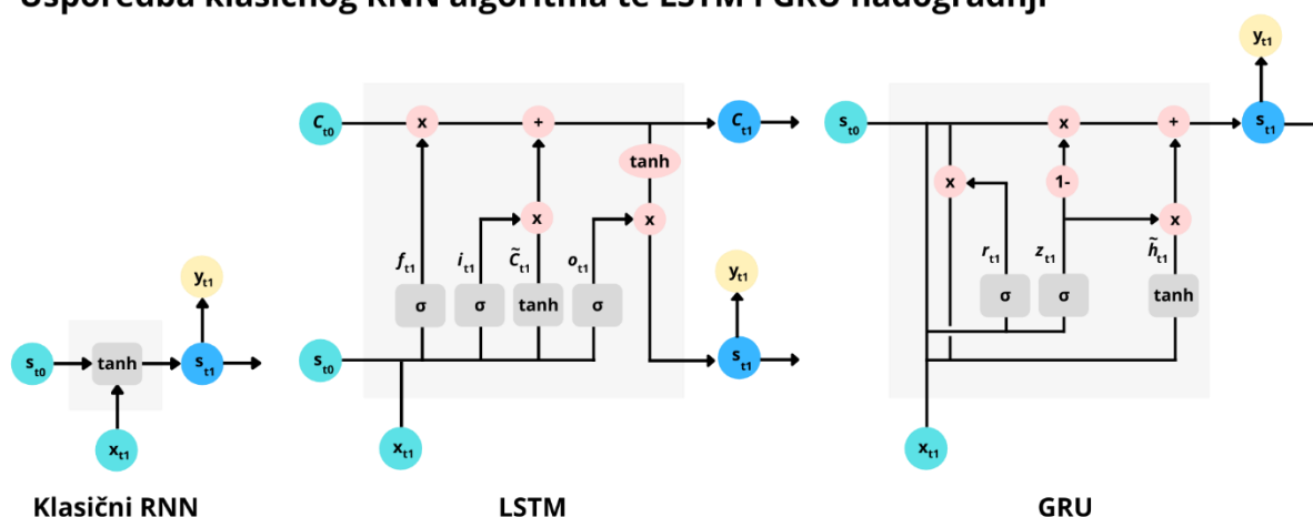
Slika 27. Usporedna klasičnog RNN algoritma te LSTM i GRU nadogradnji; prilagođeno od Aslam et al. [53]
