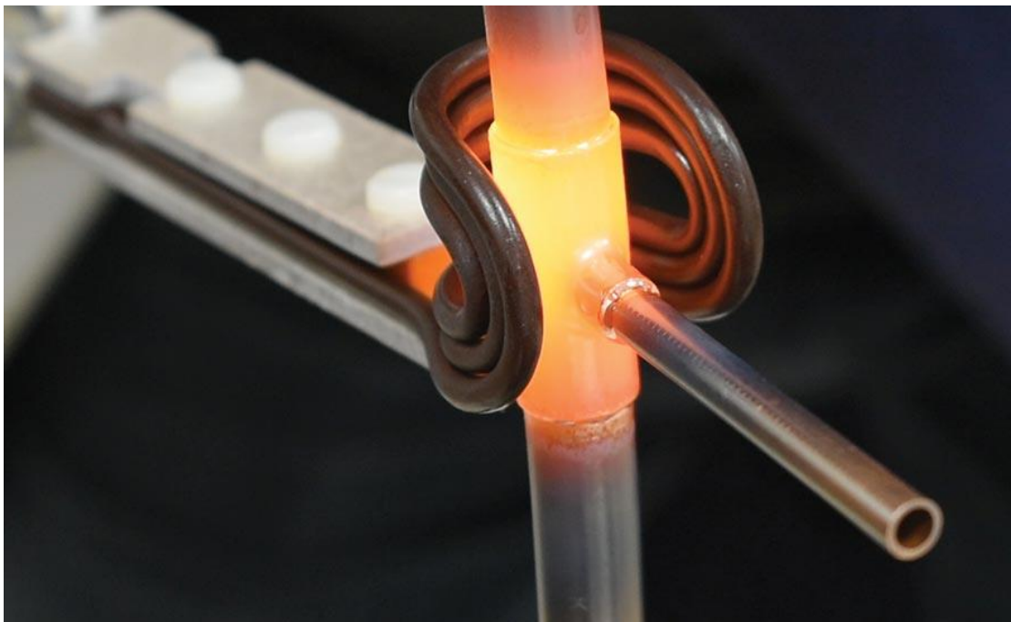
Slika 21 Induktivno lemljenje [22]
