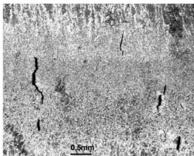
Slika 19. Nastanak hladnih pukotina prilikom mokrog podvodnog zavarivanja [1]
