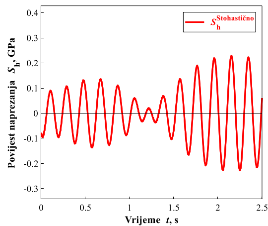
Slika 6.16 Dio povijesti napreznja za f_1 = 5\text{Hz} , f_2 = 100\text{Hz} , S_{PSD1} = 10000 \text{ MPa}^2/\text{Hz} , S_{PSD2} = 2,5 \text{ MPa}^2/\text{Hz}
