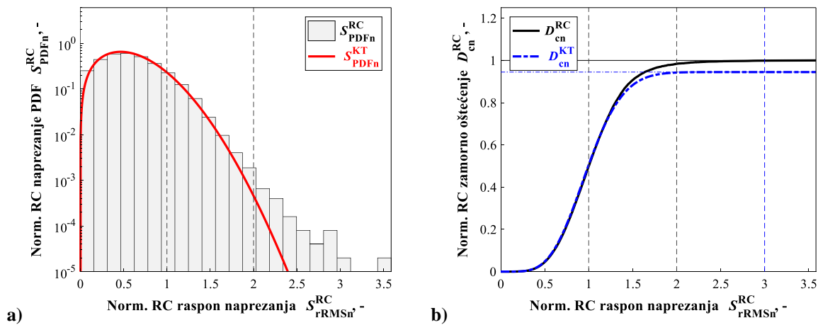
Slika 6.12 RC metoda a) PDF dijagram naprezanja b) dijagram zamornog oštećenja
