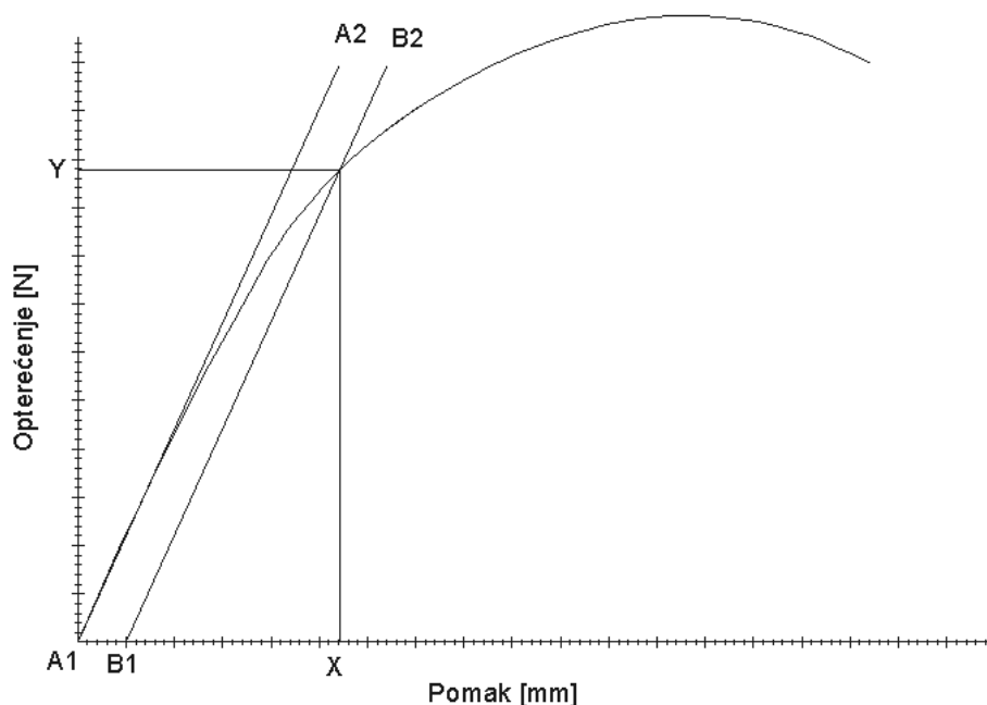
Slika 3.2 Dijagram opterećenje/pomak
