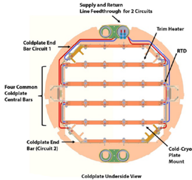
Slika 2.4: Prikaz isparivača [4]
