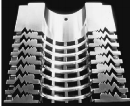
Slika 1.10: Zupčasti trim [3]
