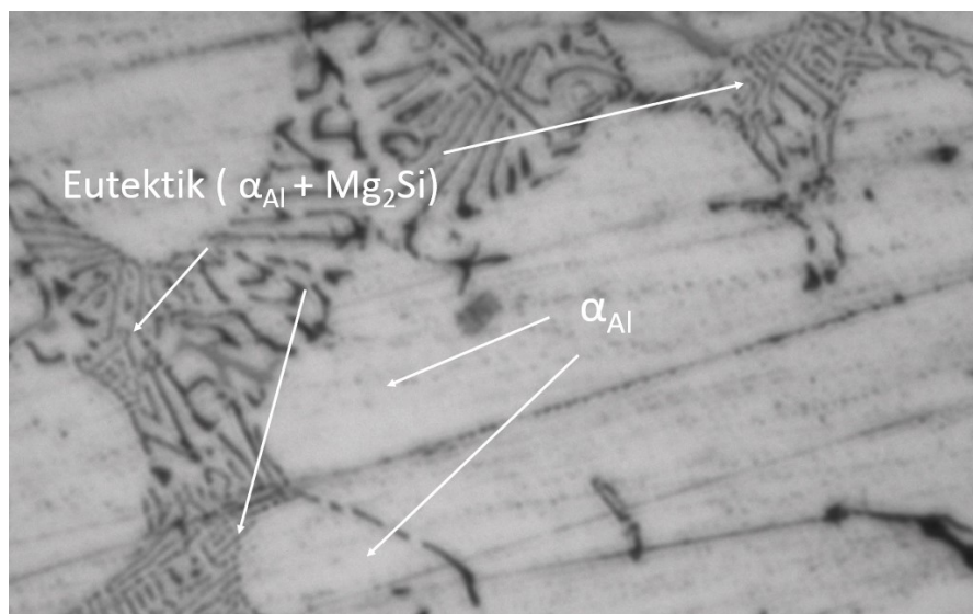
Slika 32. Pretpostavljene glavne mikrostrukturne faze
