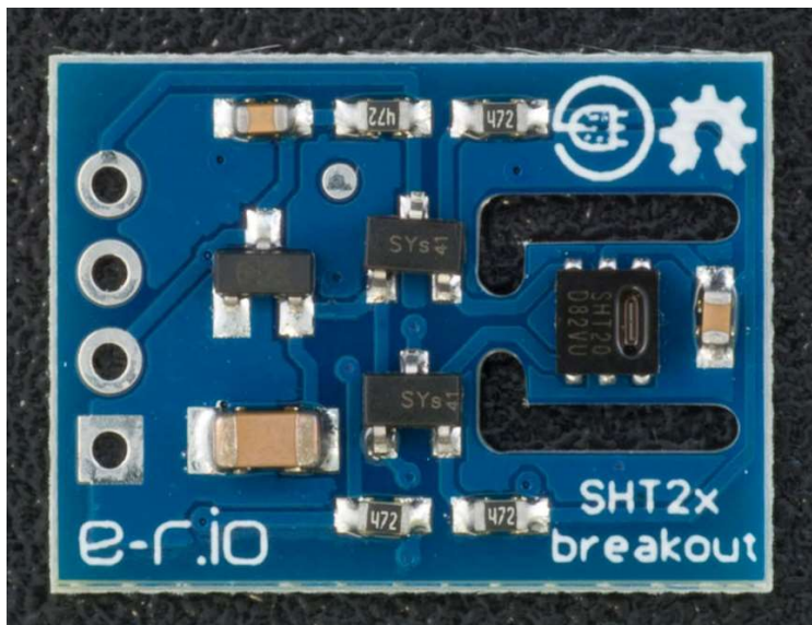
Slika 3.3. SHT20 senzor temperature i vlage
