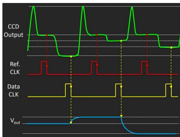
Slika 10. CDS CCD senzora [17]
