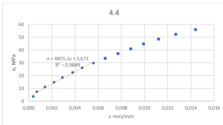
Slika 38. Krivulja naprežanje-istežanje za ispitno tijelo 4.4
