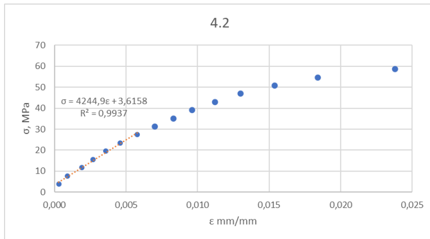
Slika 36. Krivulja naprežanje-istežanje za ispitno tijelo 4.2
