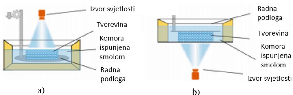
Slika 4.13. Izvedbe 3D pisača MSLA: a) bottom-up , b) top-down [25]
