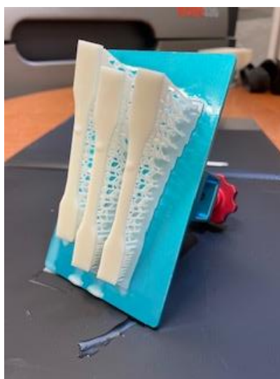
Slika 5.5. Radna podloga pisača s 3 proizvedena ispitna tijela
