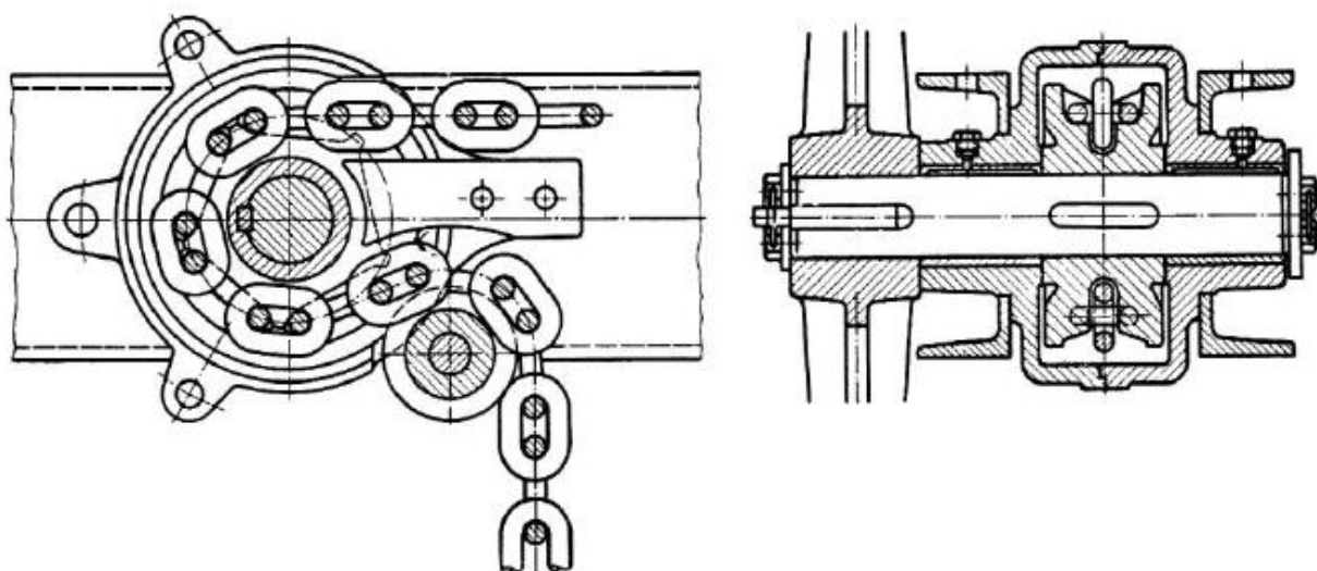
Slika 55 Vođenje lanca [10]
