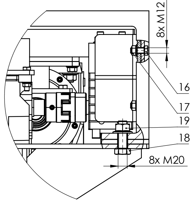
Detalj C M 1:5
