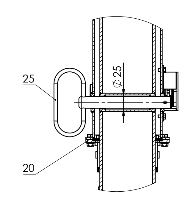
Detalj E M 1:5
