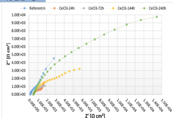
Slika 95. Nyquistov prikaz EIS eksperimentalnih vrijednosti inhibiranih i neinhibiranih uzoraka (lijevo); numeričke vrijednosti oksidnog sloja/filma inhibitora, otpora oksidnog sloja/filma inhibitora i kapaciteta električnog dvosloja (desno) nakon uranjanja u aeriranu 10 mM vodenu otopinu bez inhibitora i s inhibitorom (4 mM)
