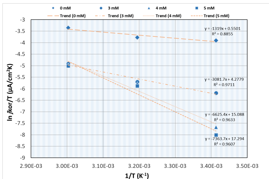
Slika 105. Grafički prikaz ovisnosti korozijskih parametara ( \ln j_{kor}/T ) i temperature ispitivanja ( (20 \pm 2) , (40 \pm 2) i (60 \pm 2) °C) uzoraka uranjenih u aeriranu 10 mM vodenu otopinu NaCl bez inhibitora i s različitim koncentracijama inhibitora (3 mM, 4 mM i 5 mM)
