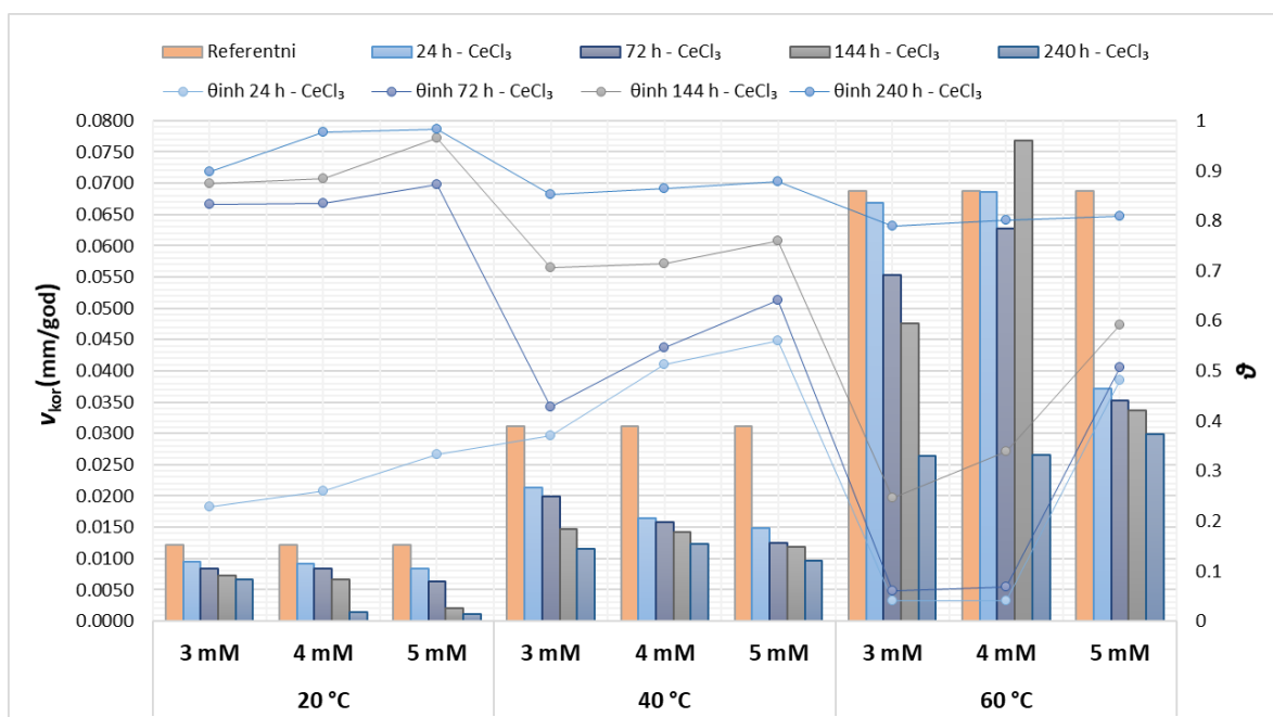
Slika 78. Grafički prikaz utjecaja ključnih varijabla na korozijsku postojanost aluminijske legure 2024-T3 nakon uranjanja u aeriranu 10 mM vodenu otopinu NaCl bez i sa \text{CeCl}_3 \times 7\text{H}_2\text{O} (3 → 5 mM)
