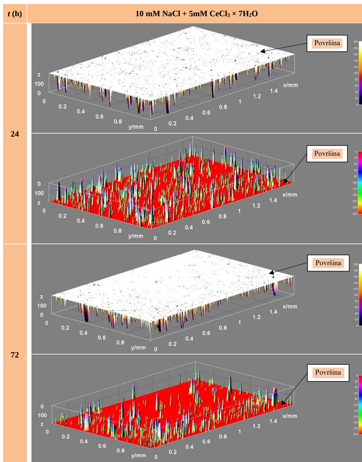
Slika 91. 3D modeli mikroskopskih jamičastih struktura nastalih kao posljedica uranjanja ispitnih uzoraka u aeriranu 10 mM vodenu otopinu NaCl sa \text{CeCl}_3 \times 7\text{H}_2\text{O} (5 mM) pri temperaturi (20 \pm 2)^\circ\text{C} i vremenskim intervalima od 24 h i 72 h
