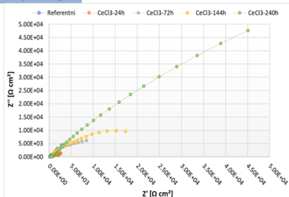
Slika 96. Nyquistov prikaz EIS eksperimentalnih vrijednosti inhibiranih i neinhibiranih uzoraka (lijevo); numeričke vrijednosti oksidnog sloja/filma inhibitora, otpora oksidnog sloja/filma inhibitora i kapaciteta električnog dvosloja (desno) nakon uranjanja u aeriranu 10 mM vodenu otopinu bez inhibitora i s inhibitorom (5 mM)
