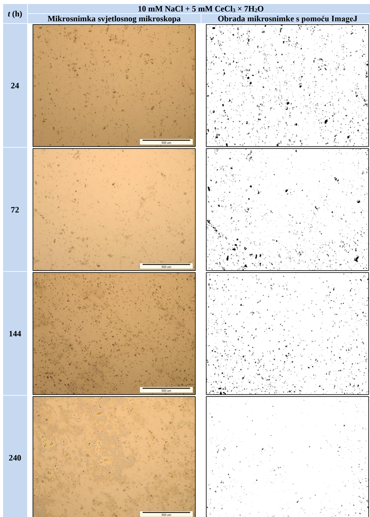
Slika 88. Mikroskopski snimci jamičastih oštećenja nastalih kao posljedica uranjanja ispitnih uzoraka u aerirano 10 mM vodenu otopinu NaCl s inhibitorom \text{CeCl}_3 \times 7\text{H}_2\text{O} (5 mM) i obrađenih s pomoću programskog paketa ImageJ (povećanje 100×)
