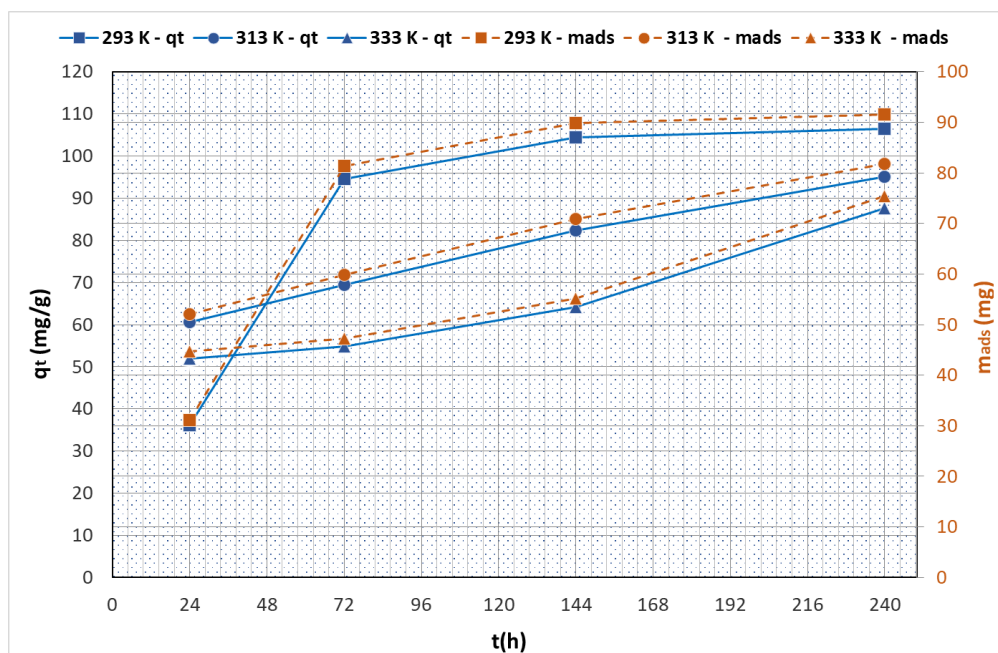
Slika 110. Grafički prikaz variranja adsorpcijskog kapaciteta i mase adsorbata na ispitnom uzorku s vremenskim intervalom uronjenosti u 10 mM vodenu otopinu NaCl s 5 mM inhibitora
