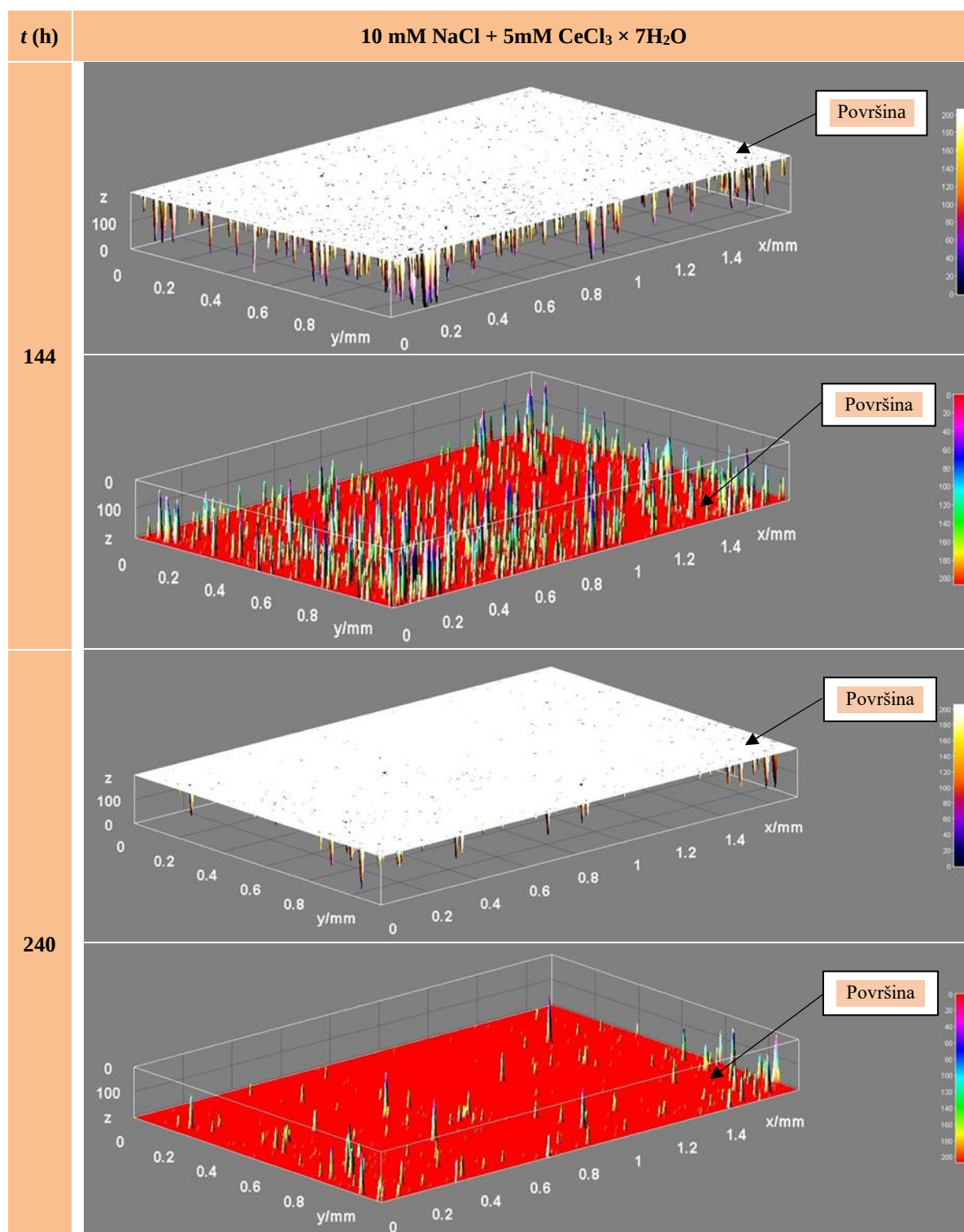
Slika 92. 3D modeli mikroskopskih jamičastih struktura nastalih kao posljedica uranjanja ispitnih uzoraka u aeriranu 10 mM vodenu otopinu NaCl sa \text{CeCl}_3 \times 7\text{H}_2\text{O} (5 mM) pri temperaturi (20 \pm 2)^\circ\text{C} i vremenskim intervalima od 144 h i 240 h
