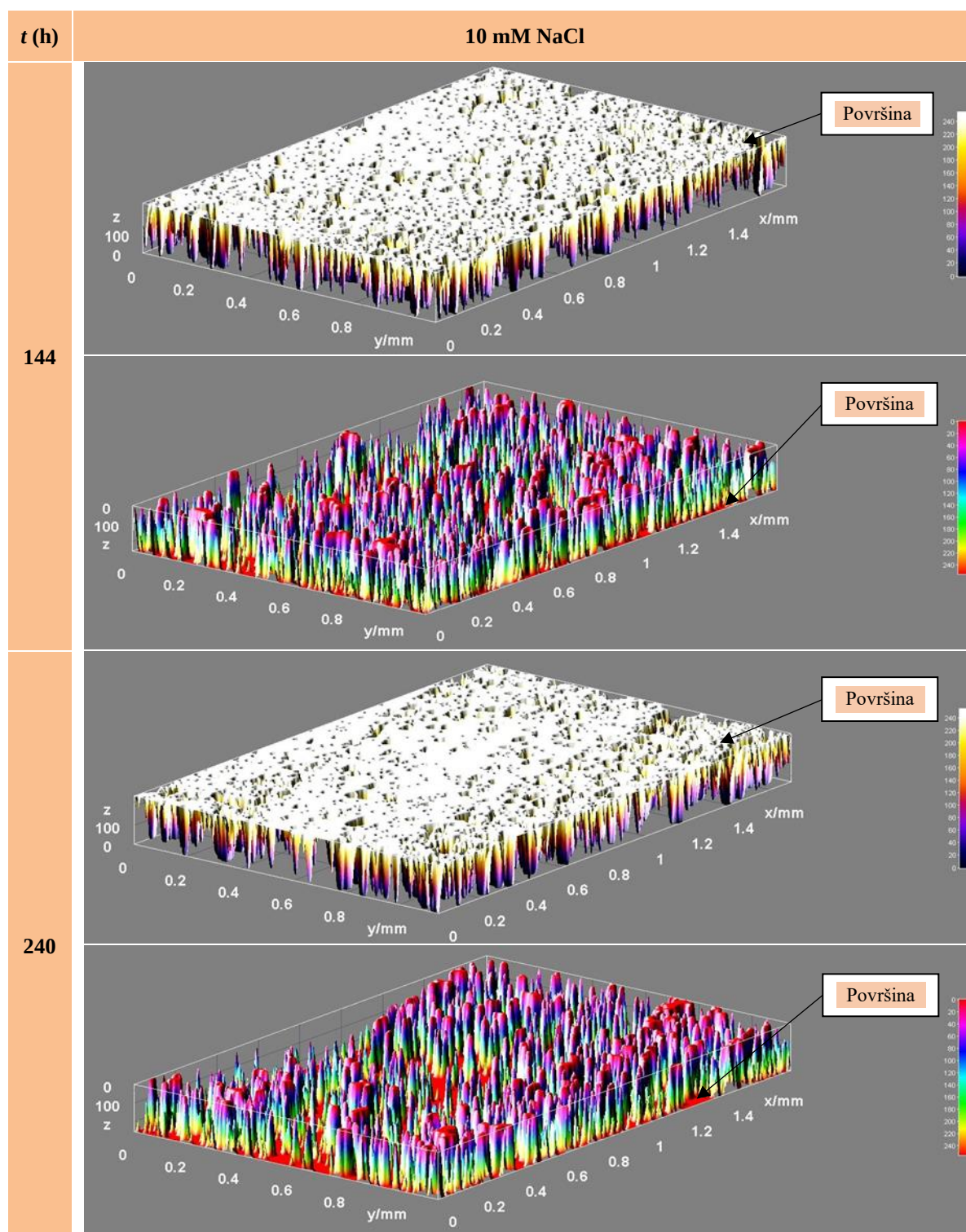
Slika 90. 3D modeli mikroskopskih jamičastih oštećenja nastalih kao posljedica uranjanja ispitnih uzoraka u aerirano 10 mM vodenu otopinu NaCl pri temperaturi (20 \pm 2) ^\circ\text{C} i vremenskim intervalima od 144 h i 240 h
