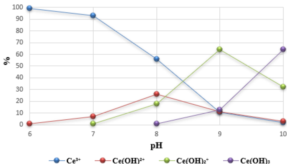
Slika 51. Postotak zastupljenosti hidroliziranih specija kao što su \text{Ce}^{3+} , \text{Ce(OH)}^{2+} , \text{Ce(OH)}_2^+ , \text{Ce(OH)}_3 i \text{Ce(OH)}_4^+ u ovisnosti o pH-vrijednosti vode [168]
