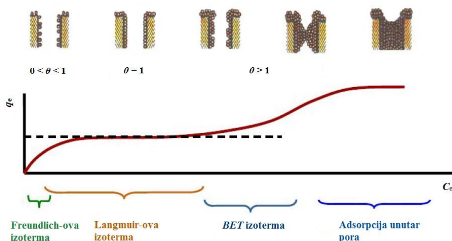
Slika 58. Prikaz najčešćih adsorpcijskih izoterma i ovisnosti q_e/C_e [205]
