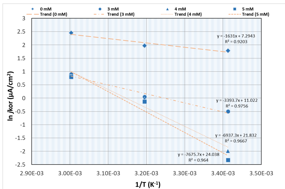
Slika 103. Grafički prikaz ovisnosti korozijskih parametara ( \ln j_{kor} ) vs. 1/T ( (20 \pm 2) , (40 \pm 2) i (60 \pm 2) °C) uzoraka uranjenih u aeriranu 10 mM vodenu otopinu NaCl bez inhibitora i s različitim koncentracijama inhibitora (3 mM, 4 mM i 5 mM)
