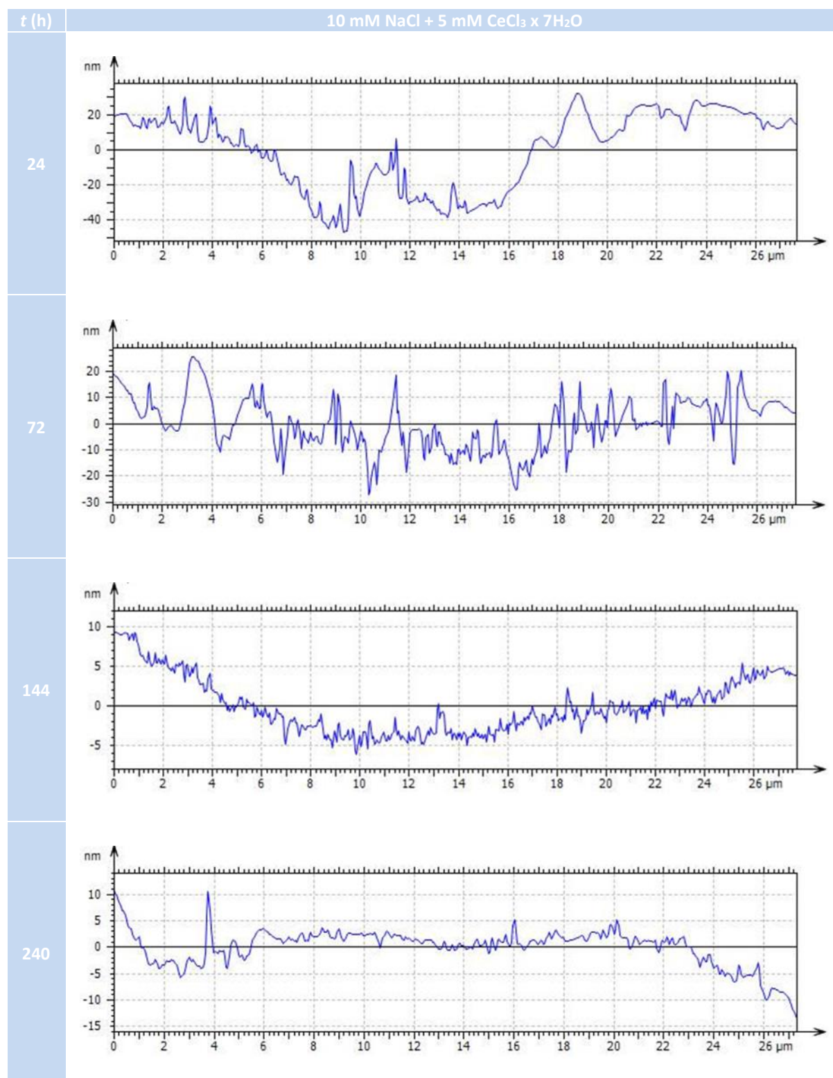
Slika 102. Prikaz linijskih profila na dijagonalama skeniranih uzoraka uronjenih u aeriranu 10 mM vodenu otopinu NaCl s (5 mM) \text{CeCl}_3 \times 7\text{H}_2\text{O} pri temperaturi od (20 \pm 2)^\circ\text{C}
