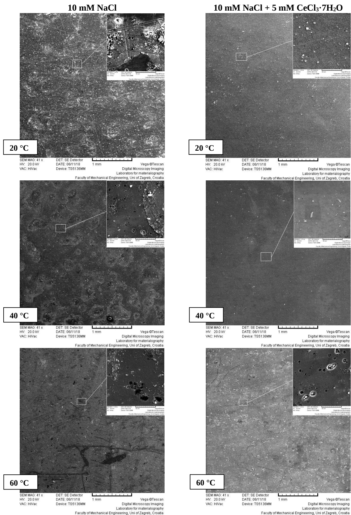
Slika 86. FE-SEM snimke površina ispitnih uzoraka uronjenih u 10 mM otopinu NaCl bez inhibitora i s inhibitorom u vremenskom periodu od 240 h i temperaturi (20 \pm 2)^\circ\text{C} , (40 \pm 2)^\circ\text{C} i (60 \pm 2)^\circ\text{C}
