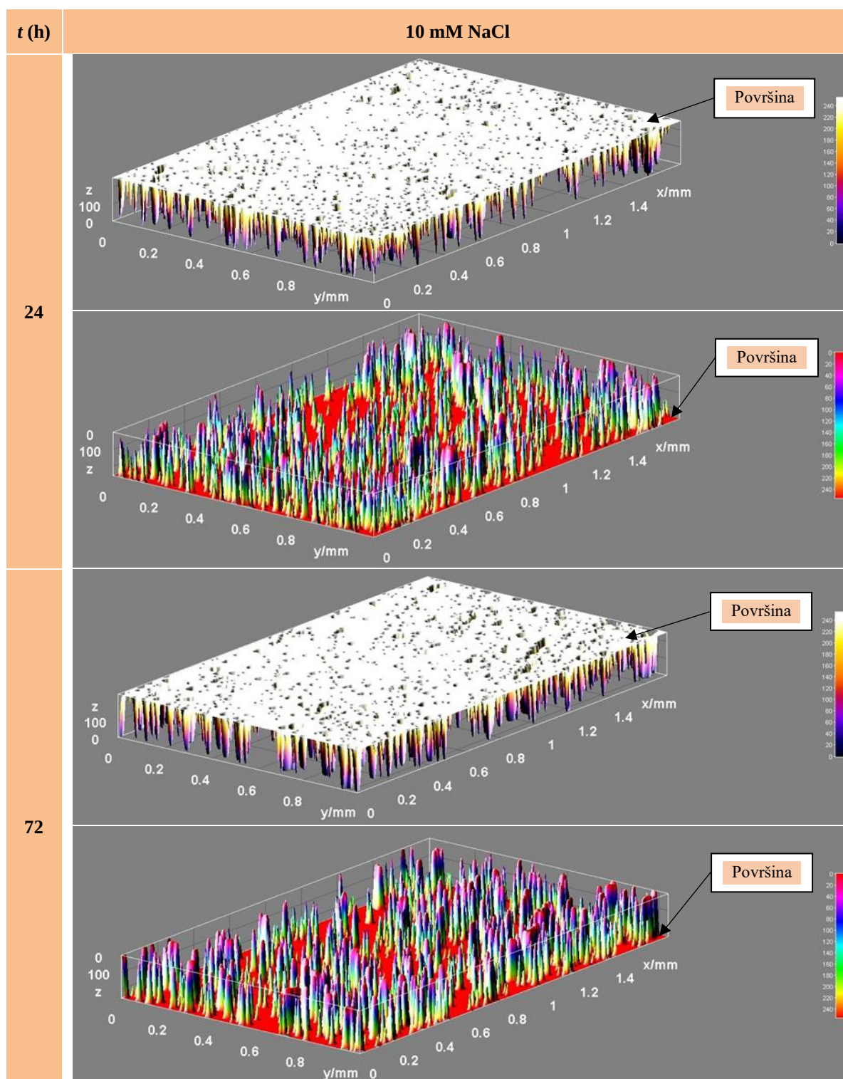
Slika 89. 3D modeli mikroskopskih jamičastih oštećenja nastalih kao posljedica uranjanja ispitnih uzoraka u aeriranu 10 mM vodenu otopinu NaCl pri temperaturi (20 \pm 2) ^\circ\text{C} i vremenskim intervalima od 24 h i 72 h
