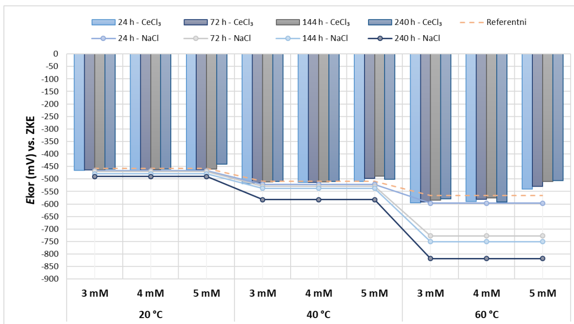
Slika 77. Grafički prikaz utjecaja ključnih varijabla na korozijski potencijal aluminijske legure 2024-T3 nakon uranjanja u aeriranu 10 mM vodenu otopinu NaCl bez i sa \text{CeCl}_3 \times 7\text{H}_2\text{O} (3 → 5 mM)
