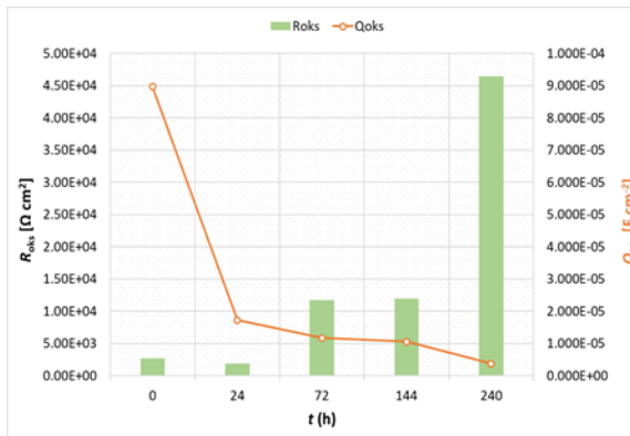
Slika 96. Nyquistov prikaz EIS eksperimentalnih vrijednosti inhibiranih i neinhibiranih uzoraka (lijevo); numeričke vrijednosti oksidnog sloja/filma inhibitora, otpora oksidnog sloja/filma inhibitora i kapaciteta električnog dvosloja (desno) nakon uranjanja u aeriranu 10 mM vodenu otopinu bez inhibitora i s inhibitorom (5 mM)
