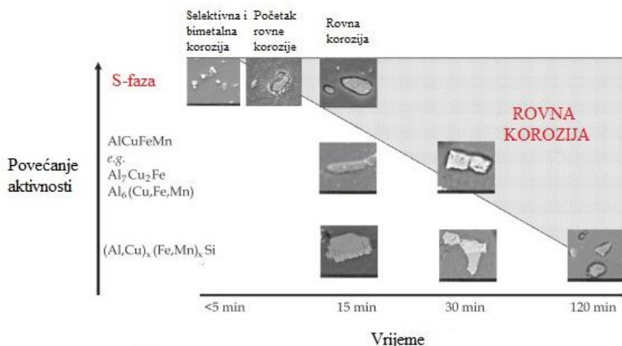
Slika 38. Slijed lokaliziranog korozijskog napada aluminijske legure 2024-T3 u kloridnom mediju [11]
