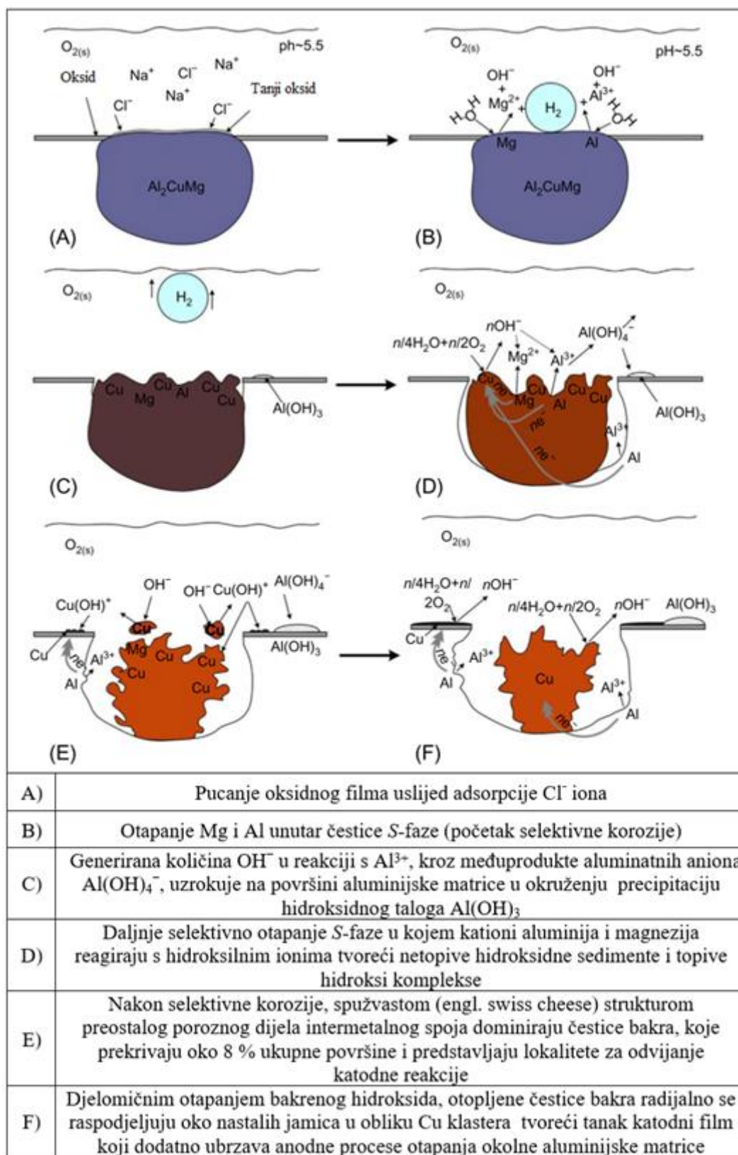
Slika 41. Shematski prikaz mehanizma nastanka jamičastih fenomena na aluminijskoj leguri 2024-T3 u kloridnom mediju: (A) pucanje oksidnog filma, (B-D) selektivna korozija S-faze, (E, F) ponovno taloženje bakra [67]
