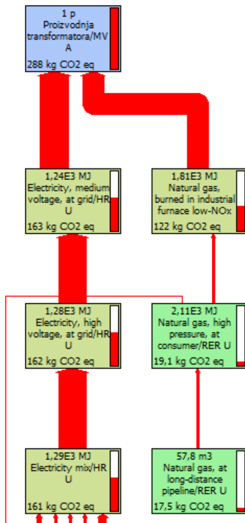
Slika 39. Ekvivalentan iznos generacije CO 2 po utrošenim resursima
