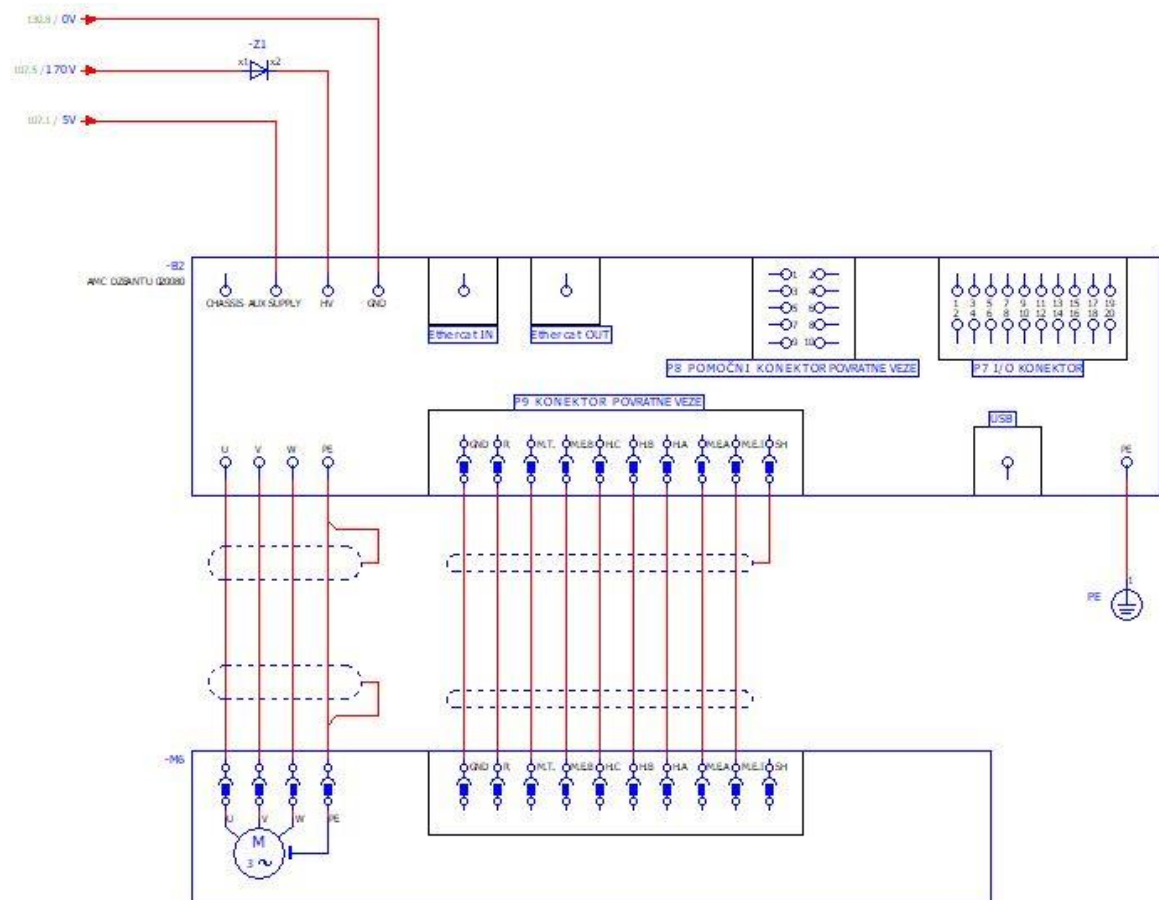
Slika 25. Regulator ekstrudera
