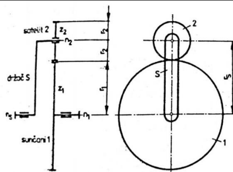
Slika 46. Jednostavni planetarni prijenosnik [16]
