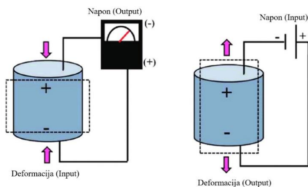
Slika 37. Prikaz piezoeфекта [24]
