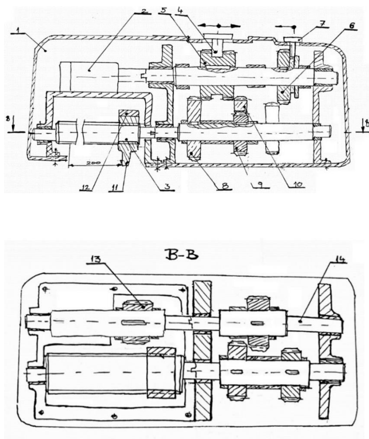
Slika 11. Skica gornjeg sklopa koncepta 1
