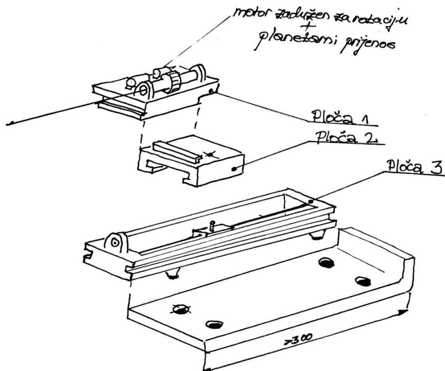
Slika 22. Skica druge verzije koncepta 4
