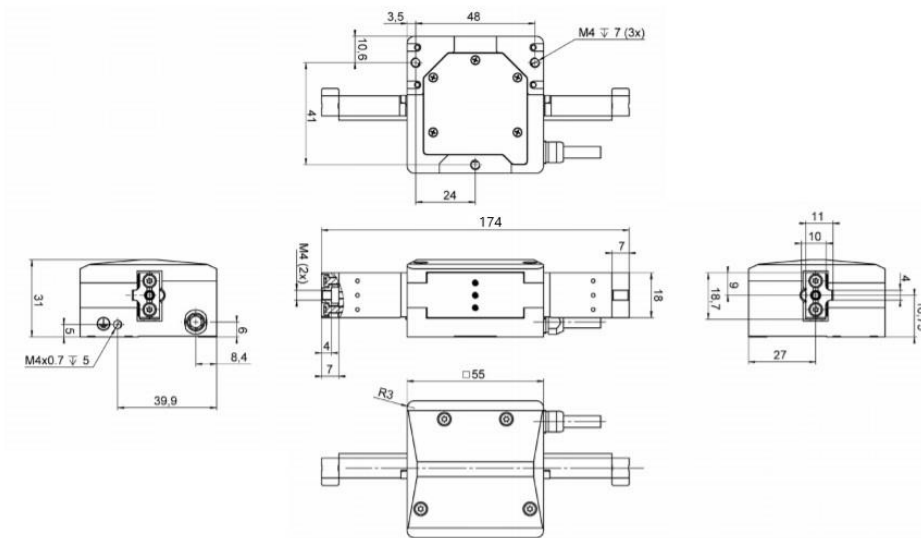
Slika 40. Prikaz dimenzija proizvoda N-331
