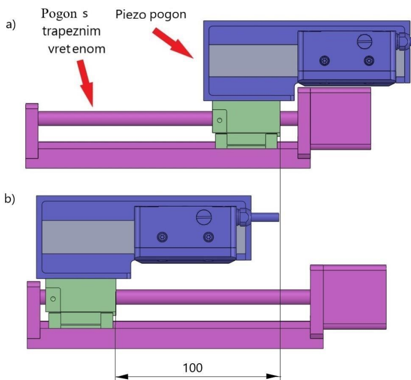
Slika 78. prikaz hoda FSL pogona a) početni položaj b) krajnji položaj
