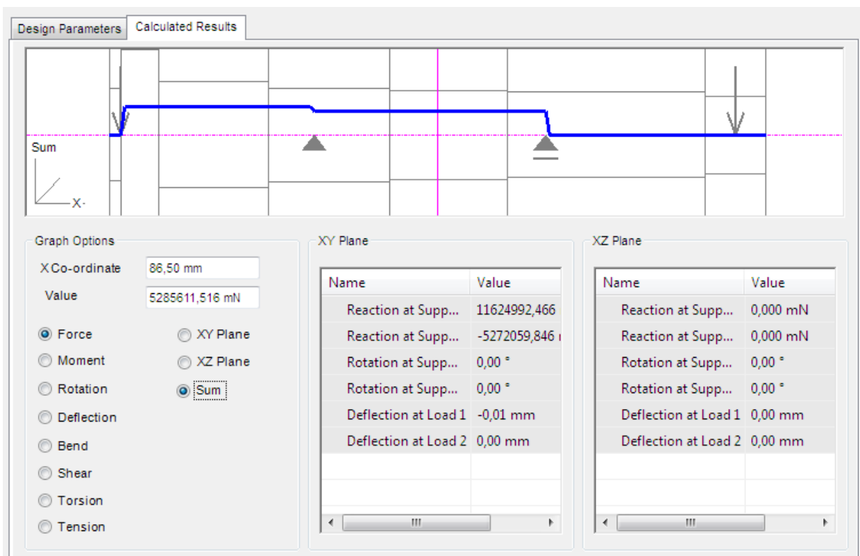
Slika 59: Dijagram sila
