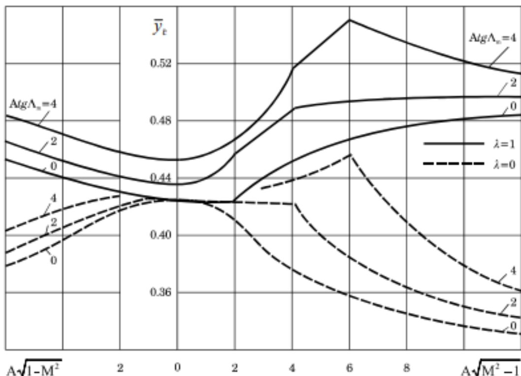
Slika 4.2 Položaj napadne točke normalne sile polu krila: \lambda=0 i \lambda=1 [6]
