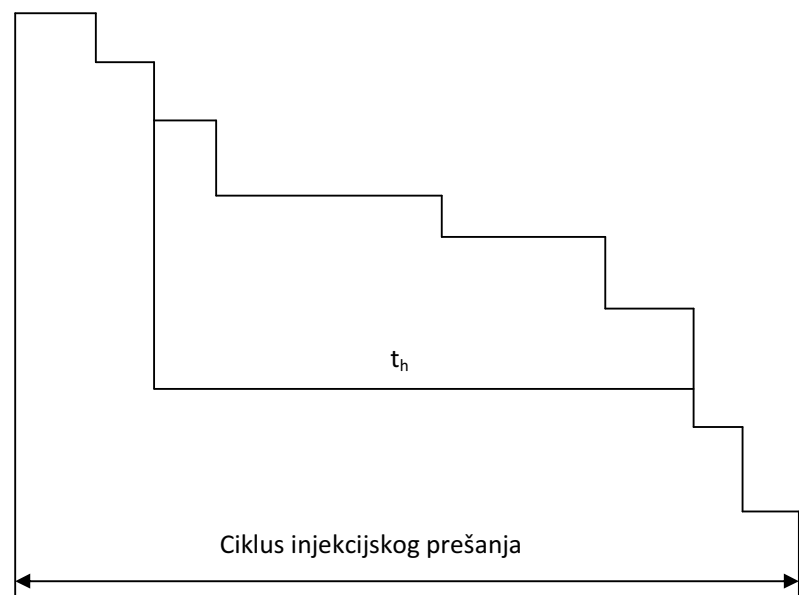
Slika 3.13. Faze ciklusa injekcijskog prešanja plastomera 9
